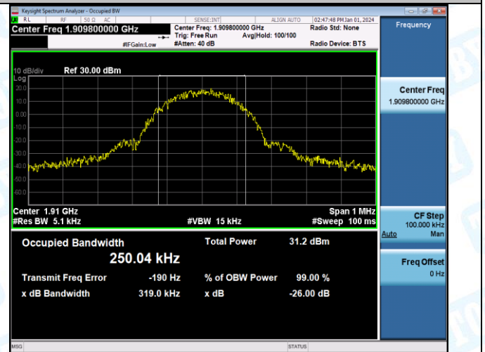
EGPRS1900-810-2-PASS
