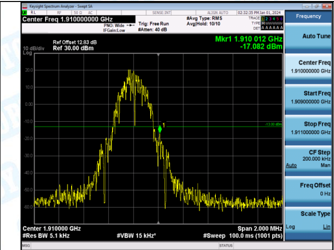
EGPRS1900-810-2-PASS
