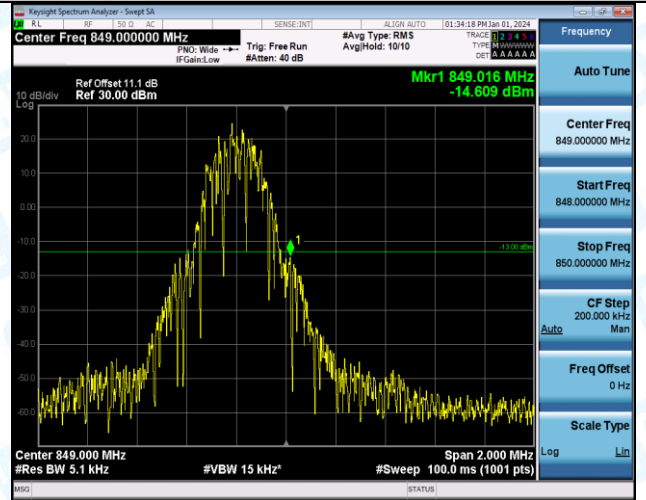
EGPRS850-251-8-PASS
