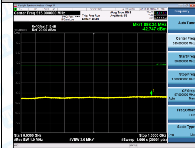
EGPRS850-190-8-30~1000MHz-PASS
