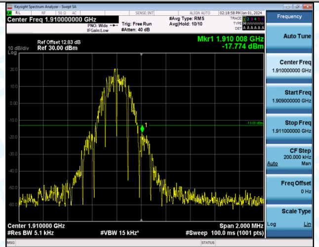
GPRS1900-810-0-PASS
