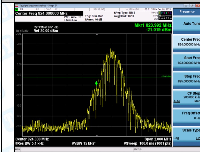
GPRS850-128-5-PASS
