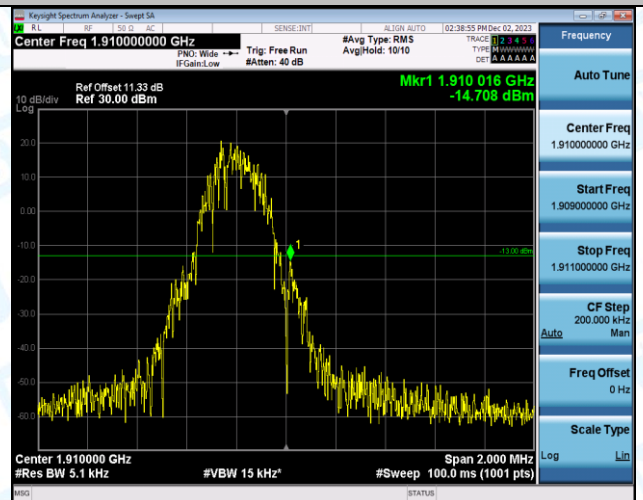
EGPRS1900-810-2-PASS
