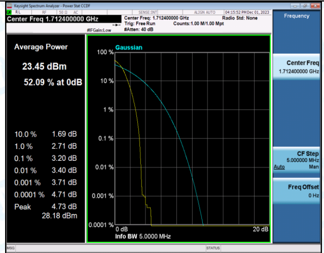
Band4-1513-PASS
