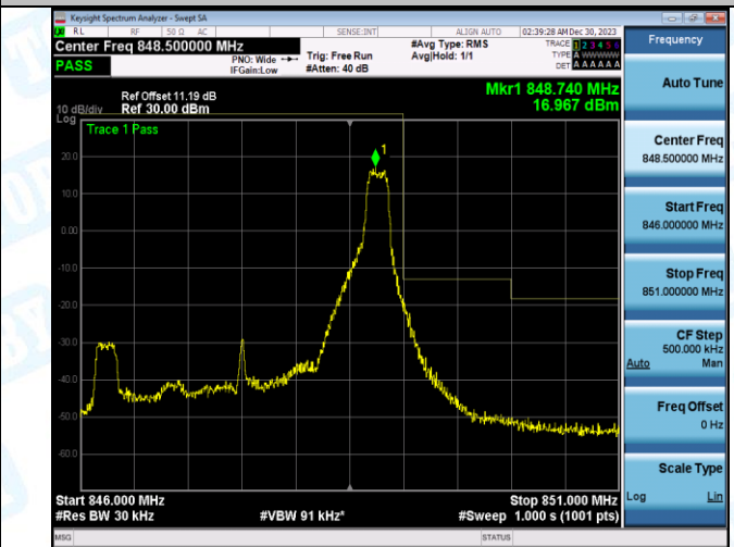
Band5_3MHz_16QAM_20635_15RB#0
