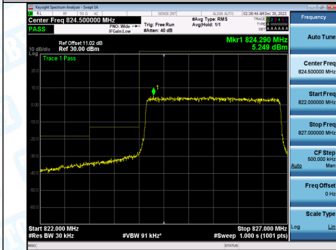
Band5_3MHz_QPSK_20635_1RB#0
