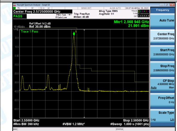
Band7_20MHz_16QAM_21350_100RB#0
