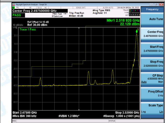
Band7_20MHz_16QAM_20850_100RB#0
