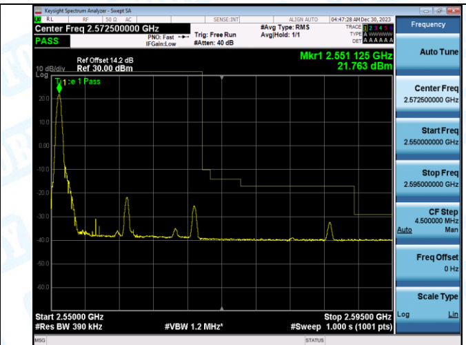
Band7_20MHz_16QAM_21350_1RB#99
