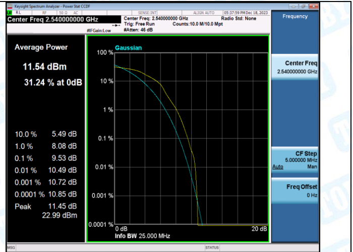
41(2535-2655)-10MHz-16QAM-40090-50RB#0-PASS
