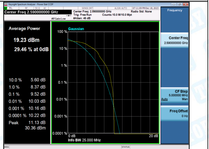
41(2535-2655)-20MHz-16QAM-40590-100RB#0-PASS
