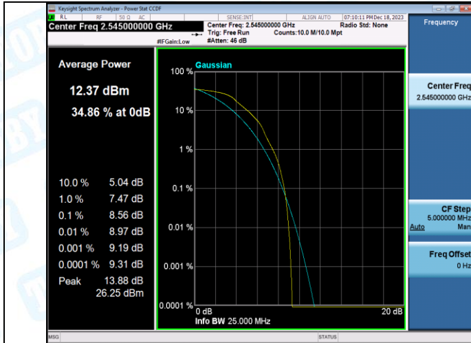
41(2535-2655)-20MHz-QPSK-40140-100RB#0-PASS
