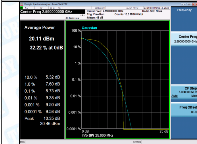
41(2535-2655)-20MHz-QPSK-40590-100RB#0-PASS
