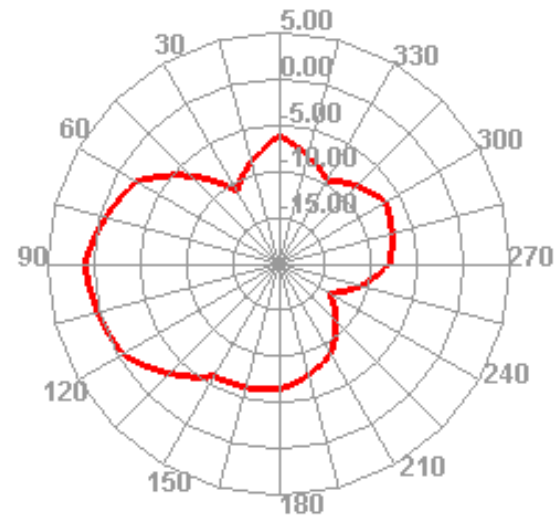
2400.000MHz E2
