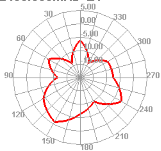
2400.000MHz E1
