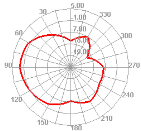
2400.000MHz H
