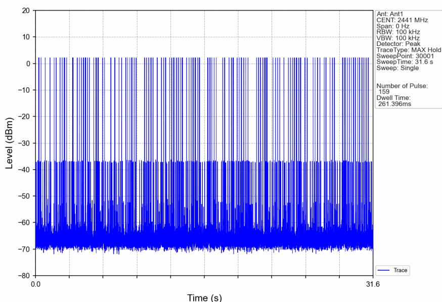
GFSK DH3 HOPP Ant1 NTNV
