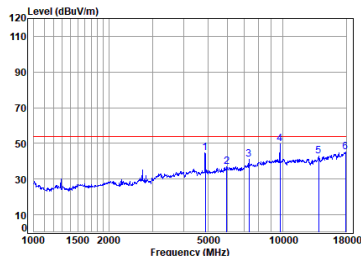
BLE_2M_TX_CH_19_Horizontal-Avg
