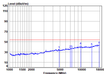
BLE_2M_TX_CH_19_Vertical-Avg
