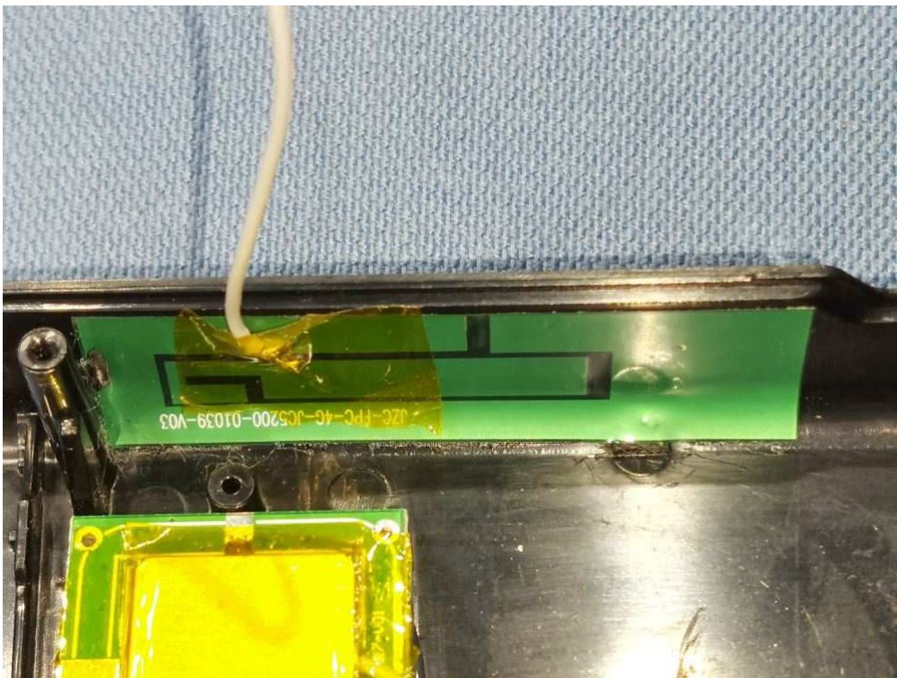
LTE Antenna
