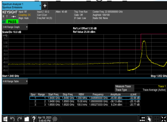
B25 1.4M 16QAM 1@0 CH 26047
