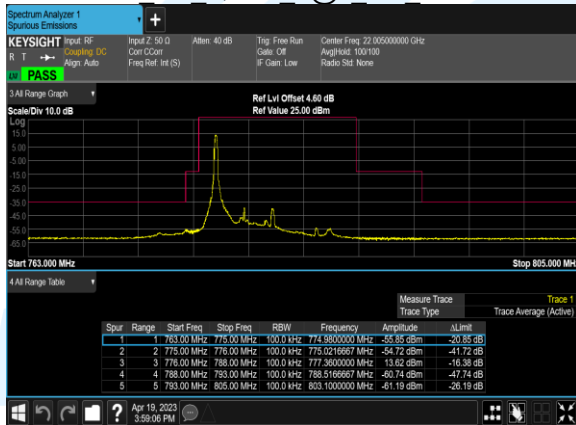
B13 5M 16QAM 1@0 CH 23205
