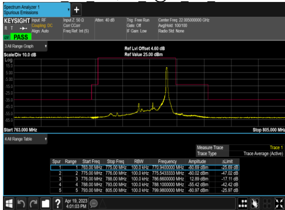
B13 5M 16QAM 1@24 CH 23255
