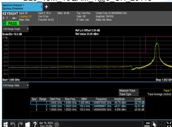
B25 15M 16QAM 1@0 CH 26115
