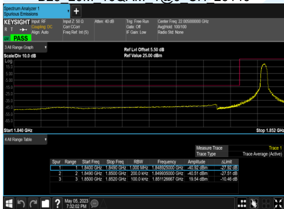
B25 20M 16QAM 1@0 CH 26140
