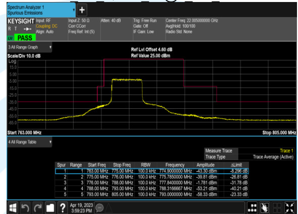
B13 5M 16QAM 25@0 CH 23205
