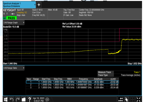
B25 5M 16QAM 25@0 CH 26065
