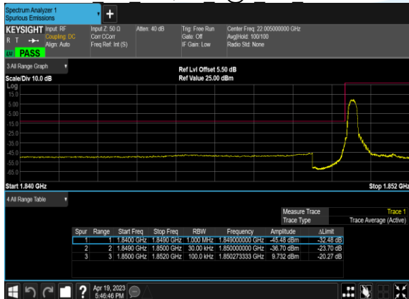
B25 3M 16QAM 1@0 CH 26055
