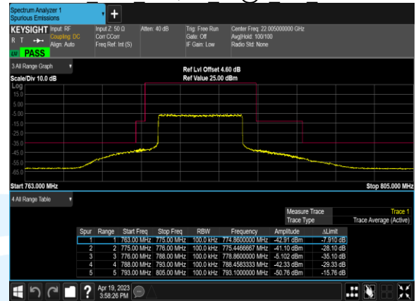
B13 5M QPSK 25@0 CH 23205
