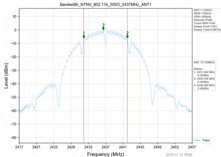
802.11b_2437MHz_SISO_ANT1
