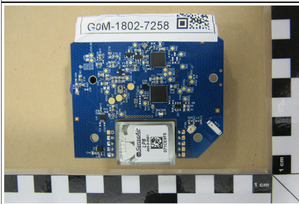
PCB Bottom
