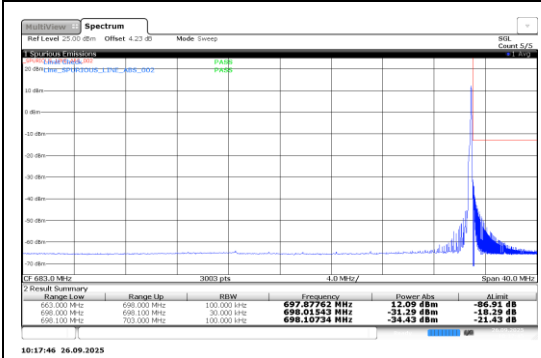
Band71-0.18-BPSK-133470-1@11-15kHz-PASS
