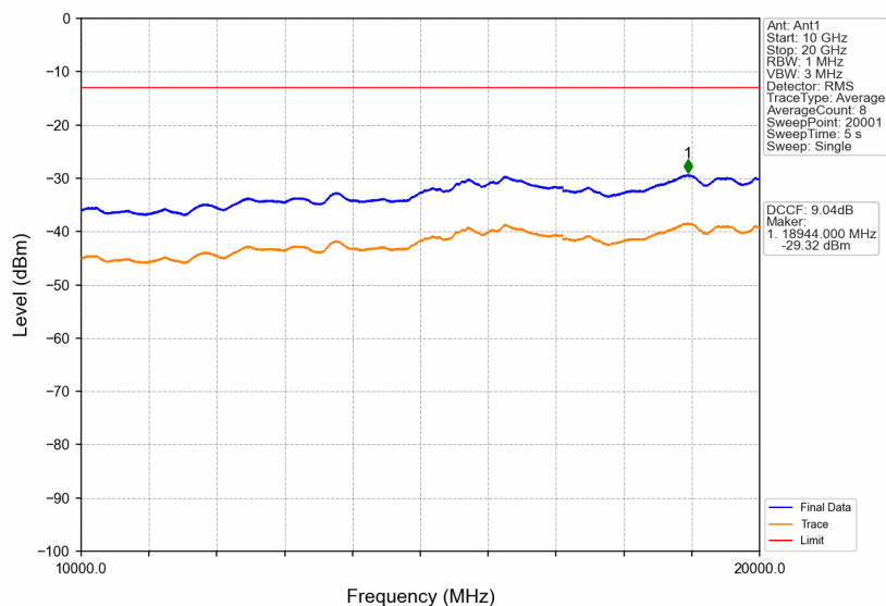
PCS1900_GSM_MCH_1880MHz_GSM_NTNV
