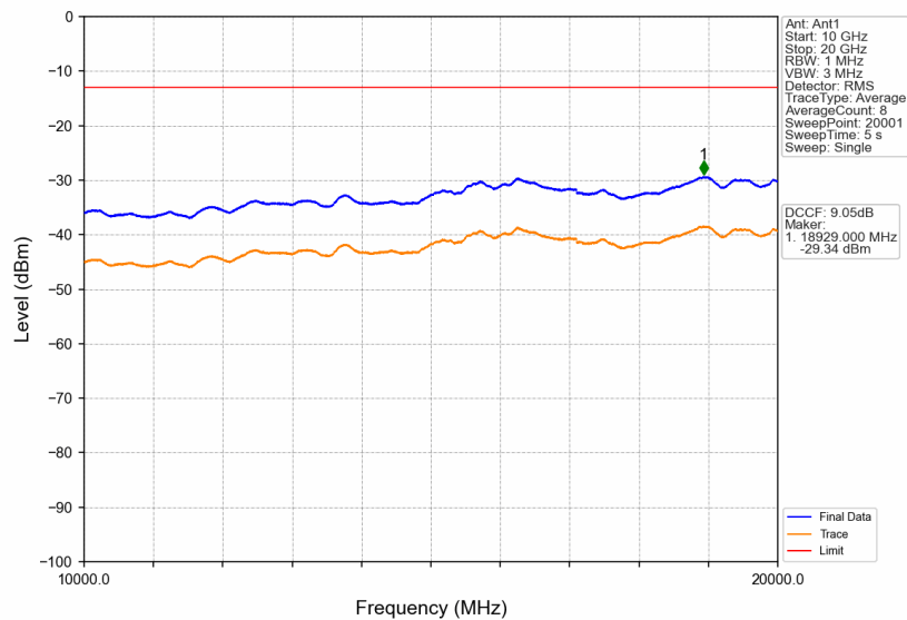
PCS1900_GSM_HCH_1909.8MHz_GSM_NTNV
