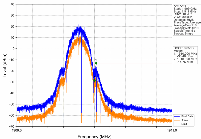
PCS1900_GSM_HCH_1909.8MHz_GSM_NTNV
