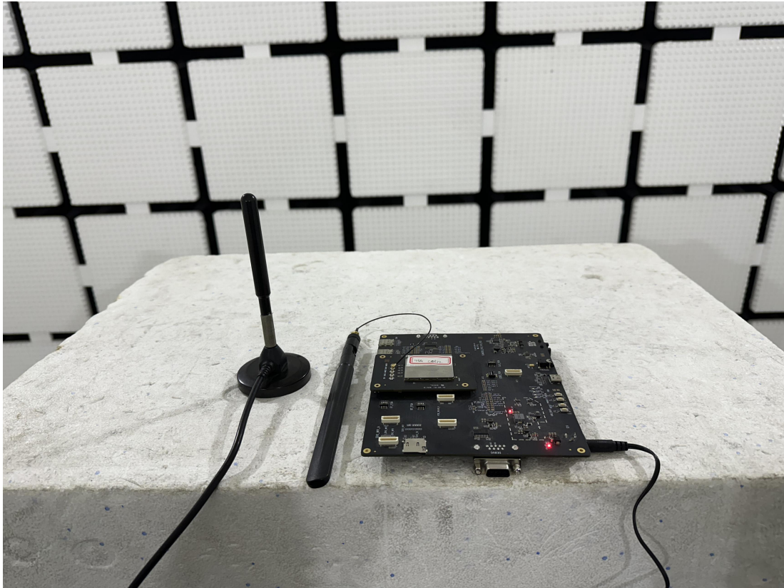
Close-up-RF
