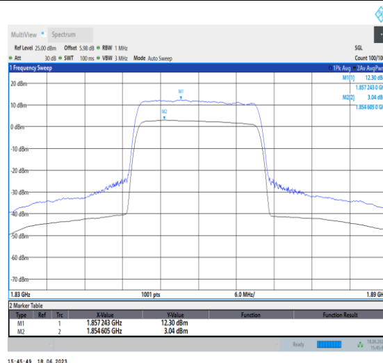
1-N2-PC3-15-20-L-2-CP-256QAM-Outer_Full-106@ 0-Ant3-9.26-100%-0.00-9.26-PASS-≤13
