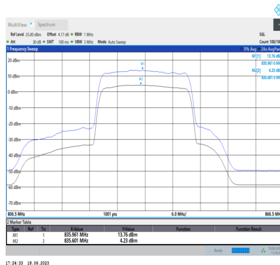
1-N5-PC3-15-20-M-2-CP-256QAM-Outet_Full-106 @0-Ant0-9.53-100%-0.00-9.53-PASS-≤13
