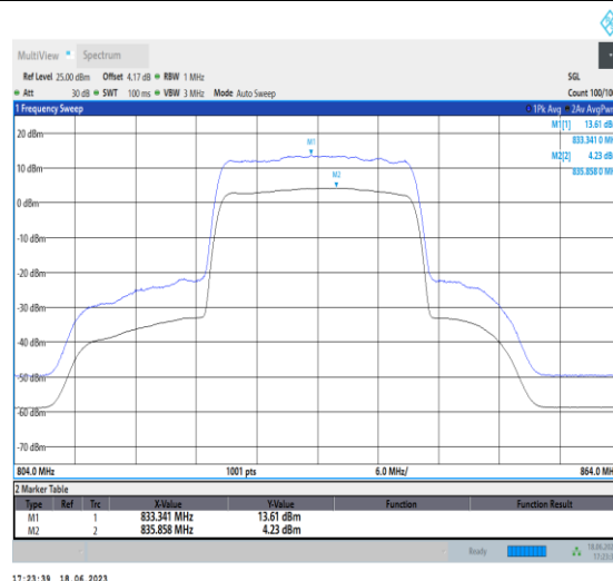
1-N5-PC3-15-20-L-2-CP-256QAM-Outet_Full-106@ 0-Ant0-9.38-100%-0.00-9.38-PASS-≤13
