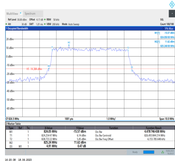
1-N5-PC3-15-5-L-4-DFT-64QAM-Outet_Full-25@0-A nt0-4.479-4.910-≤5-PASS
