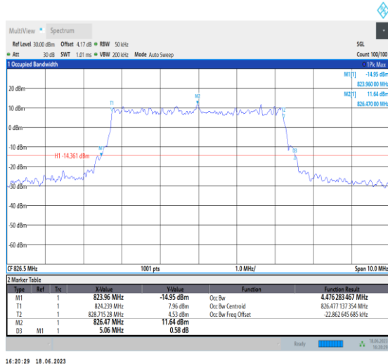
1-N5-PC3-15-5-L-3-DFT-16QAM-Outet_Full-25@0-A Ant0-4.476-5.060-≤5-PASS
