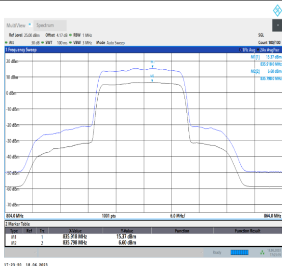
1-N5-PC3-15-20-L-1-DFT-256QAM-Outet_Full-100@ 0-Ant0-8.77-100%-0.00-8.77-PASS-≤13
