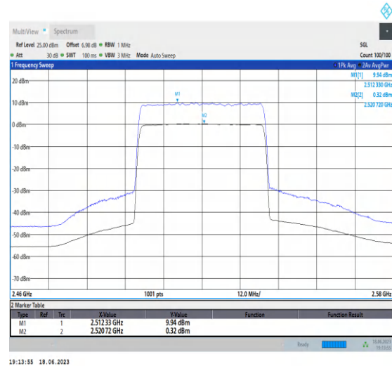
1-N7-PC3-15-40-L-2-CP-256QAM-Outter_Full-216@ 0-Ant0-9.62-100%-0.00-9.62-PASS-≤13
