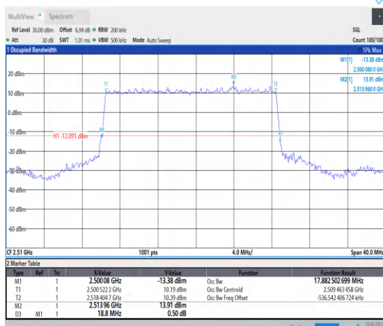
1-N7-PC3-15-20-L-2-DFT-PI2BPSK-Outer_Full-100@0-Ant0-17.883-18.800-≤20-PASS
