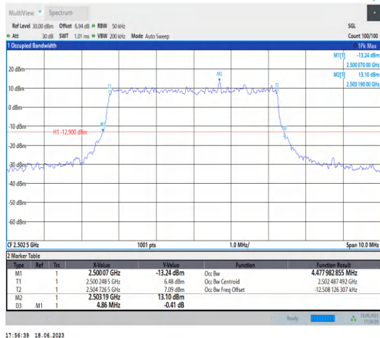
1-N7-PC3-15-5-L-1-DFT-QPSK-Outer_Full-25@0-An t0-4.478-4.860-≤5-PASS
