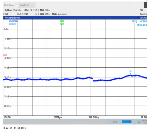
1-N38-PC2-30-40-L-1-N/A-DFT-QPSK-Edge_1RB_L eft-1@0-12000-20000-Ant0-18964.00--47.19--25-PA SS
