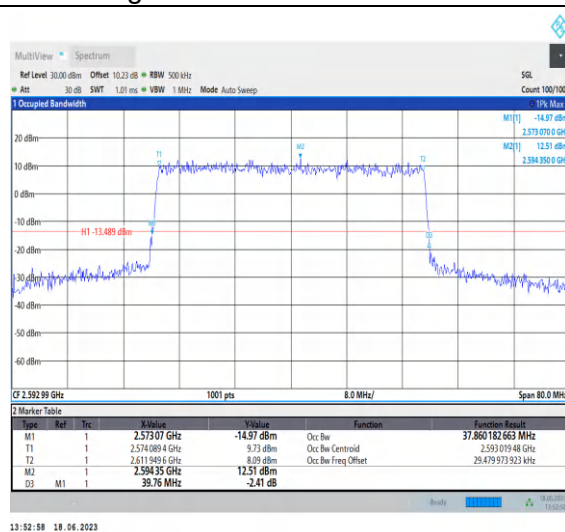
1-N41-PC3-30-40-M-7-CP-16QAM-Outer_Full-106@ 0-Ant0-37.86-39.760-≤40-PASS
