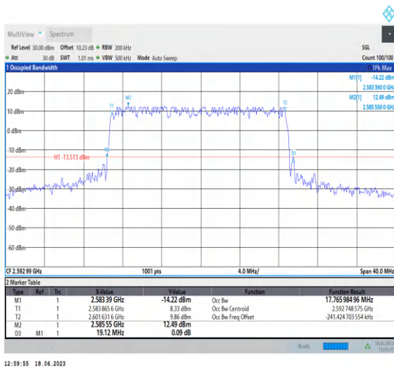
1-N41-PC3-30-20-M-2-DFT-QPSK-Outer_Full-50@0 -Ant0-17.766-19.120-≤20-PASS
