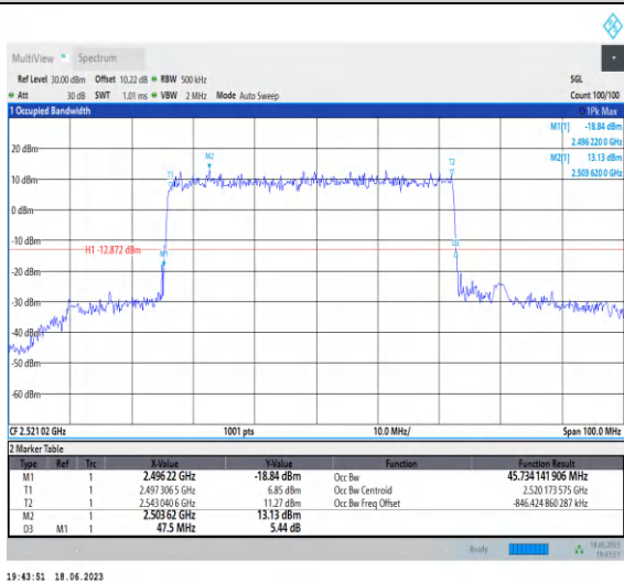
1-N41-PC3-30-50-L-2-DFT-QPSK-Outer_Full-128@ 0-Ant0-45.734-47.500-≤50-PASS
