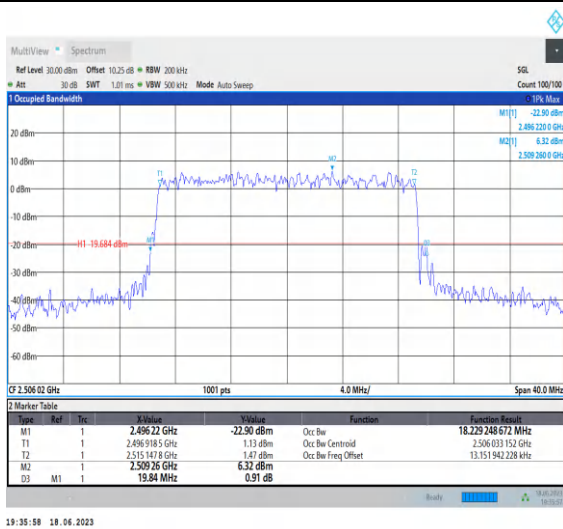
1-N41-PC3-30-20-L-9-CP-256QAM-Outer_Full-51@ 0-Ant0-18.229-19.840-≤20-PASS
