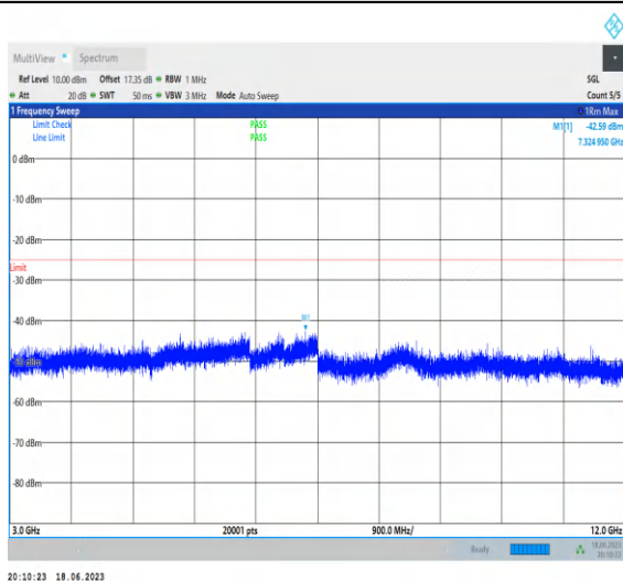
1-N41-PC3-30-100-M-1-N/A-DFT-PI2BPSK-Inner_1 RB_Left-1@1-3000-12000-Ant0-7324.95--42.59--25 -PASS
