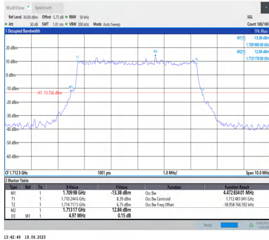
1-N66-PC3-15-5-L-1-DFT-QPSK-Outet_Full-25@0-A nt3-4.473-4.970-≤5-PASS
