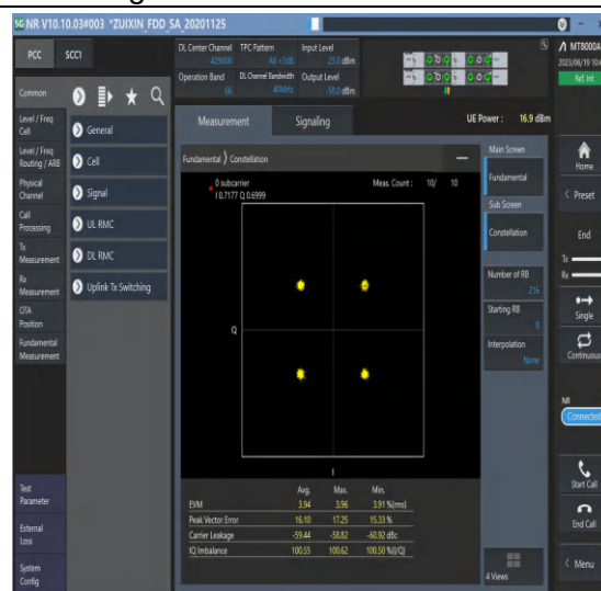
1-N66-PC3-15-40-M-6-CP-QPSK-Outer_Full-216@ 0-Ant3-see graph-PASS
