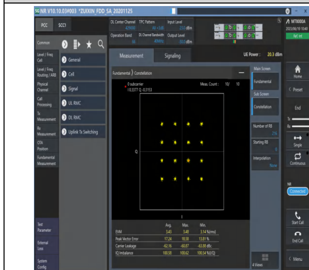
1-N66-PC3-15-40-M-7-CP-16QAM-Outer_Full-216@ 0-Ant3-see graph-PASS
