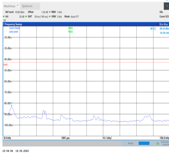
1-N66-PC3-15-40-H-1-DFT-PI2BPSK-Inner_1RB_L eft-1@1-0.009-0.15-Ant3-0.02--83.24--43-PASS
