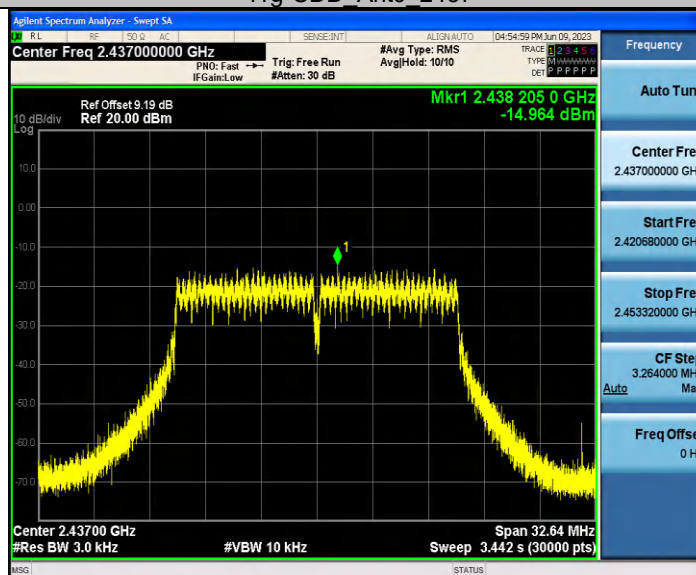
11q-CDD Ant1 2437
