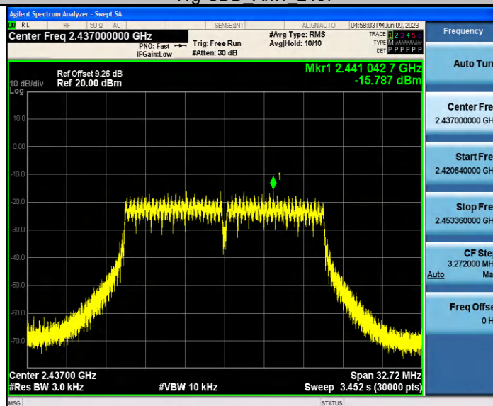
11q-CDD Ant1 2437
