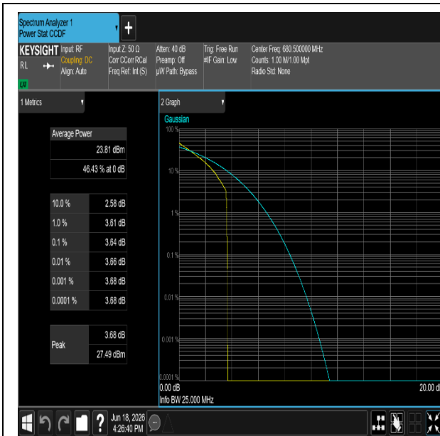
NTNV-n71-PC3-15-20-H-DFT-QPSK-Edge_1RB_Left-PASS
