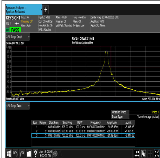
NTNV-n71-PC3-15-15-L-DFT-QPSK-Edge_1RB_Left-PASS
