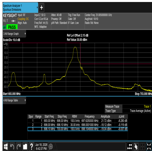
NTNV-n71-PC3-15-10-L-DFT-QPSK-Edge_1RB_Left-PASS
