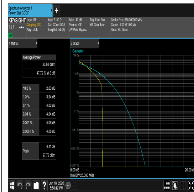
NTNV-n71-PC3-15-20-H-DFT-QPSK-Edge_1RB_Left-PASS
