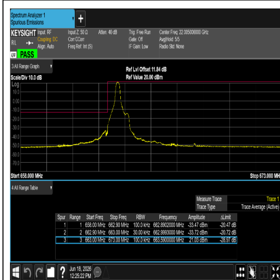
Band71-10MHz-QPSK-133172-1RB#0-PASS
