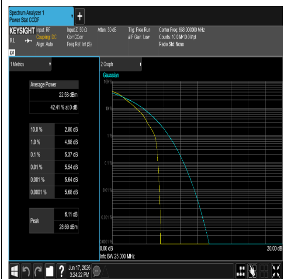
Band71-20MHz-QPSK-133372-1RB#0-PASS
