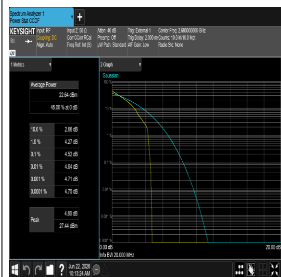
Band41-20MHz-QPSK-41490-1RB#0-PASS
