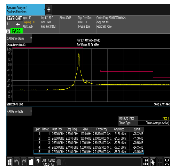
Band41-20MHz-QPSK-41490-1RB#99-PASS
