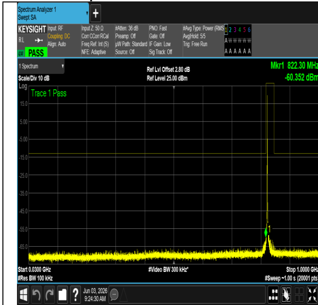
NTNV-n26(824-849)-PC3-15-20-M-DFT-QPSK- Edge 1RB Left-3000-12000-PASS
