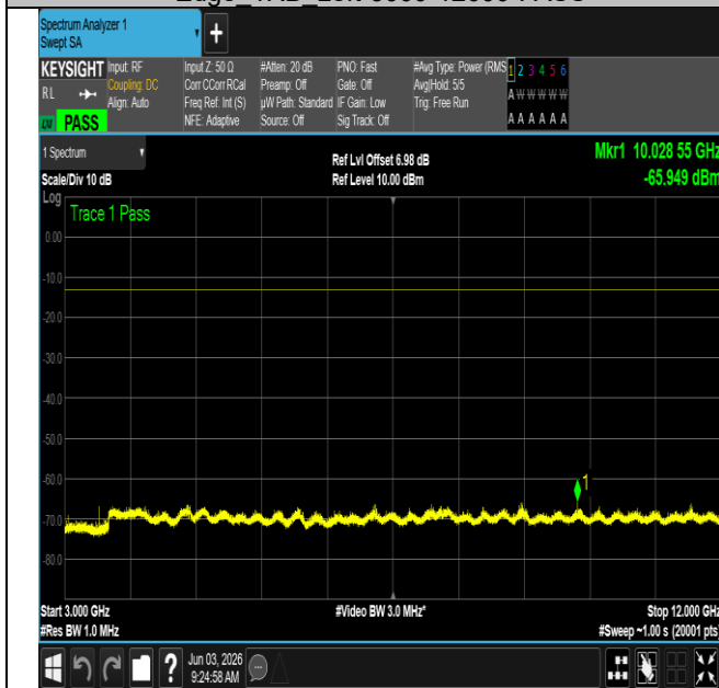
NTNV-n26(824-849)-PC3-15-20-H-DFT-QPSK- Edge 1RB Left-30-1000-PASS
