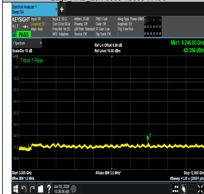
NTNV-n26(824-849)-PC3-15-20-M-DFT-QPSK-Edge 1RB Left-30-1000-PASS
