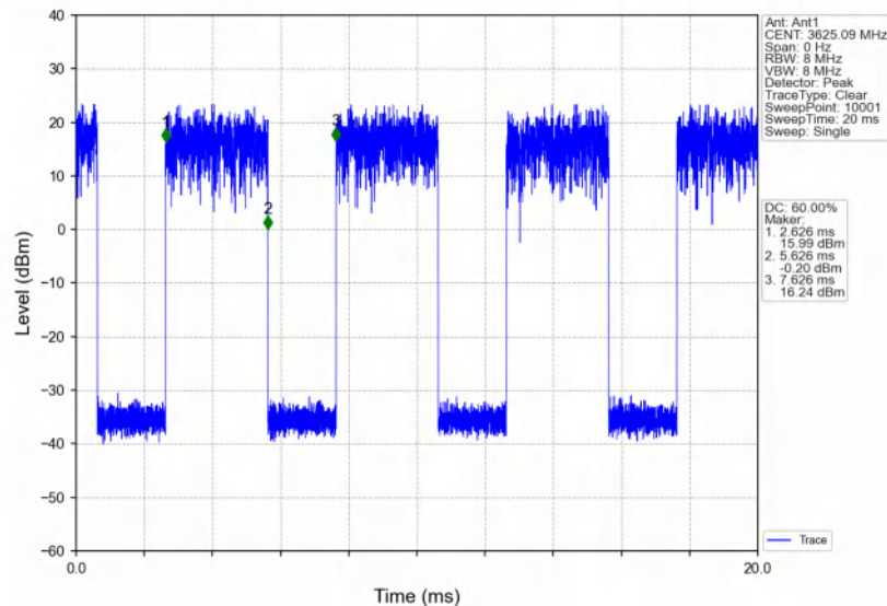
Band48_10MHz_64QAM_MCH_3625MHz_RB_1_49_NTNV
