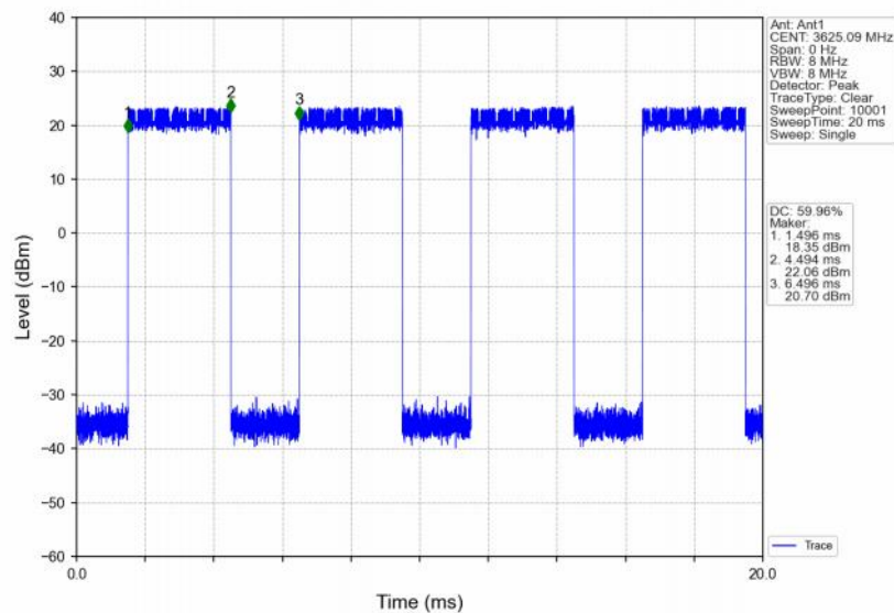
Band48_10MHz_QPSK_MCH_3625MHz_RB_25_13_NTNV
