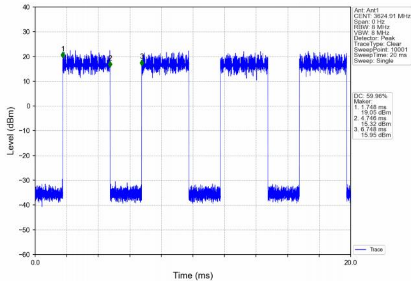
Band48_5MHz_256QAM_MCH_3625MHz_RB_12_13_NTNV
