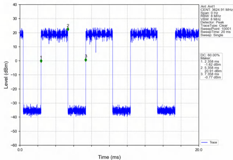
Band48_5MHz_64QAM_MCH_3625MHz_RB_12_6_NTNV
