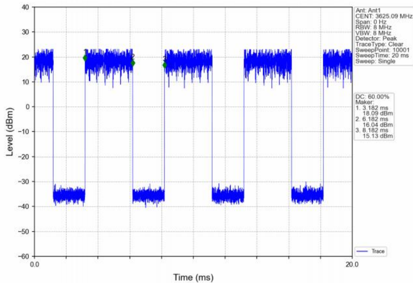
Band48_10MHz_QPSK_MCH_3625MHz_RB_1_49_NTNV
