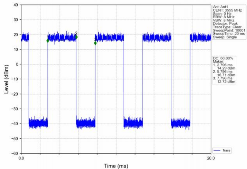
Band48_10MHz_256QAM_LCH_3555MHz_RB_50_0_NTNV
