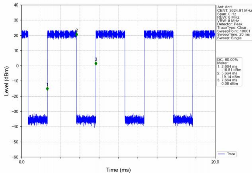
Band48_5MHz_QPSK_MCH_3625MHz_RB_12_6_NTNV
