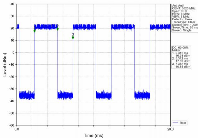
Band48_5MHz_QPSK_MCH_3625MHz_RB_25_0_NTNV
