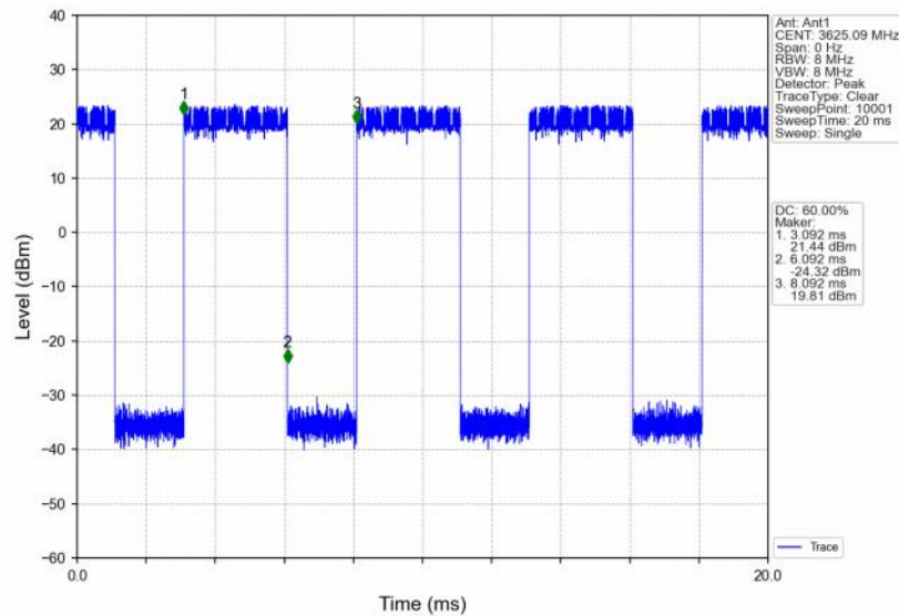
Band48_10MHz_16QAM_MCH_3625MHz_RB_25_25_NTNV
