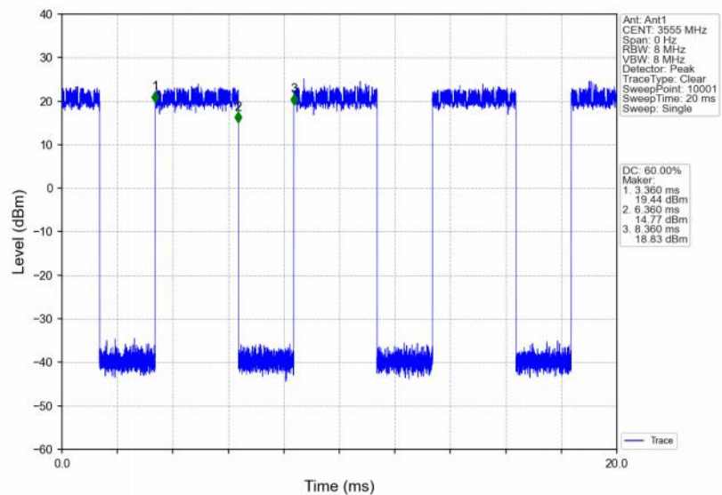
Band48_10MHz_16QAM_LCH_3555MHz_RB_50_0_NTNV
