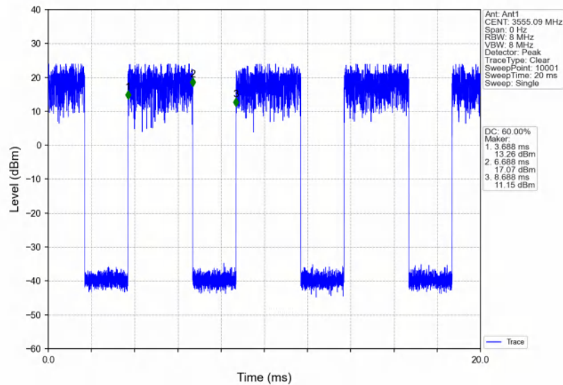
Band48_10MHz_16QAM_LCH_3555MHz_RB_1_49_NTNV
