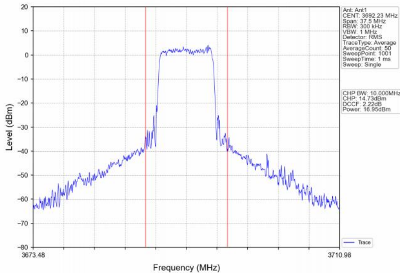
Band48_15MHz_64QAM_HCH_3692.5MHz_RB_36_39_NTNV
