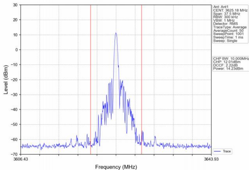
Band48_15MHz_256QAM_MCH_3625MHz_RB_1_38_NTNV
