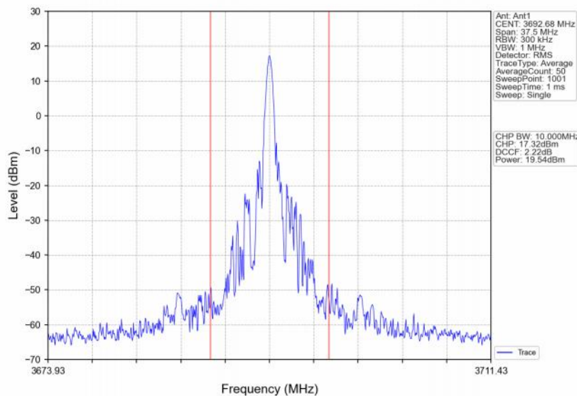
Band48_15MHz_QPSK_HCH_3692.5MHz_RB_1_38_NTNV
