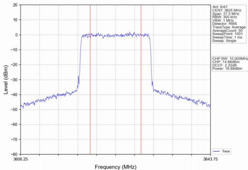
Band48_15MHz_QPSK_MCH_3625MHz_RB_75_0_NTNV
