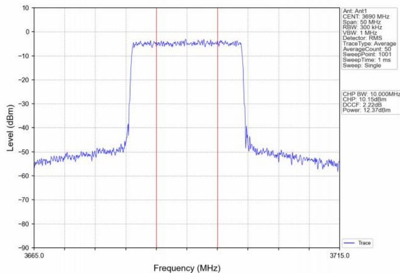
Band48_20MHz_256QAM_HCH_3690MHz_RB_100_0_NTNV
