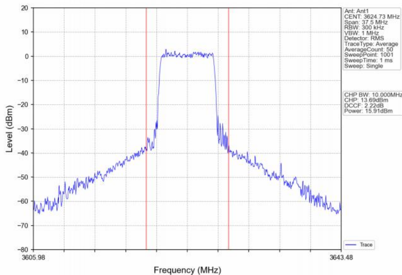
Band48_15MHz_64QAM_MCH_3625MHz_RB_36_18_NTNV
