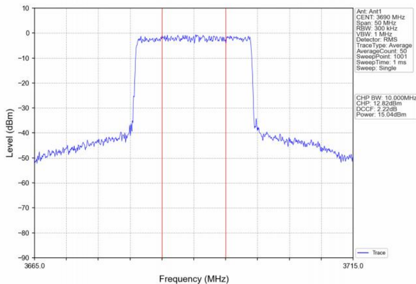
Band48_20MHz_16QAM_HCH_3690MHz_RB_100_0_NTNV
