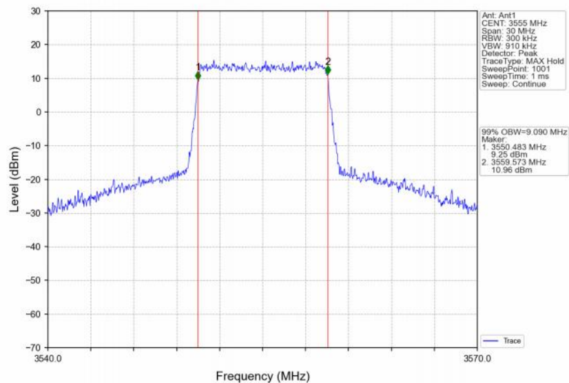
Band48_10MHz_16QAM_LCH_3555MHz_RB_50_0_NTNV
