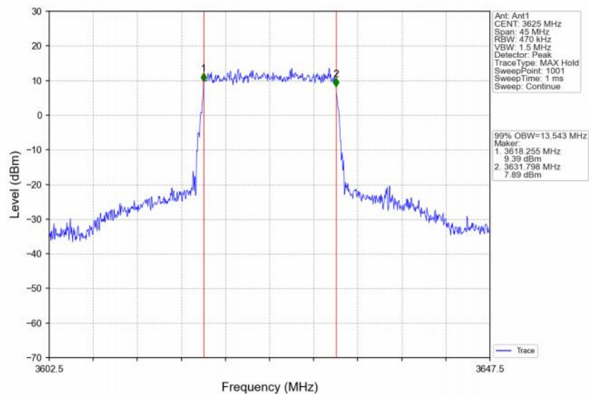
Band48_15MHz_QPSK_MCH_3625MHz_RB_75_0_NTNV
