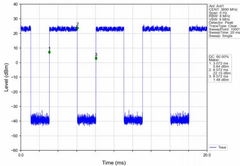
Band48_20MHz_QPSK_HCH_3690MHz_RB_50_50_NTNV
