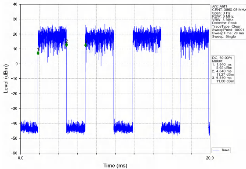
Band48_20MHz_256QAM_LCH_3560MHz_RB_1_99_NTNV
