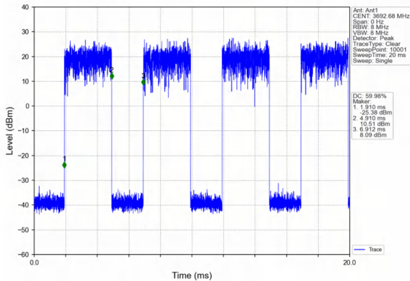
Band48_15MHz_256QAM_HCH_3692.5MHz_RB_1_74_NTNV
