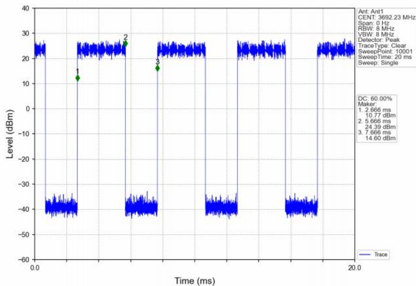
Band48_15MHz_256QAM_HCH_3692.5MHz_RB_36_18_NTNV
