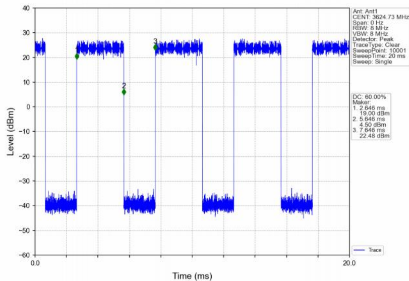
Band48_15MHz_64QAM_MCH_3625MHz_RB_36_18_NTNV
