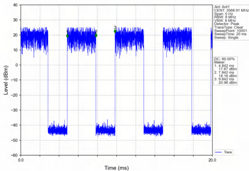
Band48_20MHz_16QAM_LCH_3560MHz_RB_1_99_NTNV
