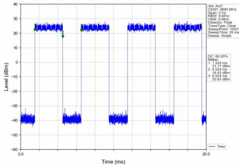
Band48_20MHz_64QAM_HCH_3690MHz_RB_50_50_NTNV
