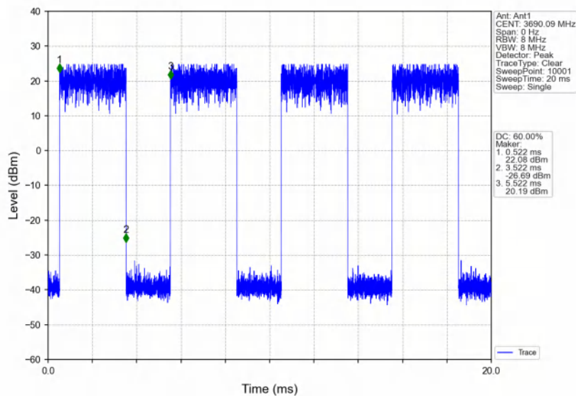
Band48_20MHz_QPSK_HCH_3690MHz_RB_1_50_NTNV
