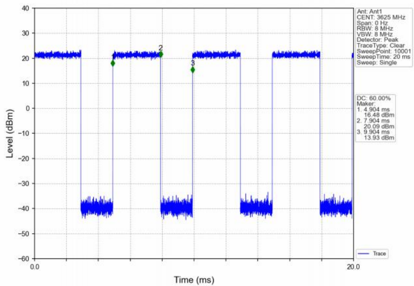
Band48_15MHz_QPSK_MCH_3625MHz_RB_75_0_NTNV
