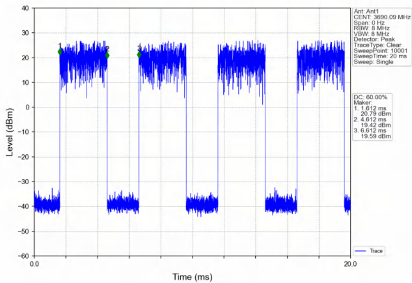
Band48_20MHz_64QAM_HCH_3690MHz_RB_1_50_NTNV
