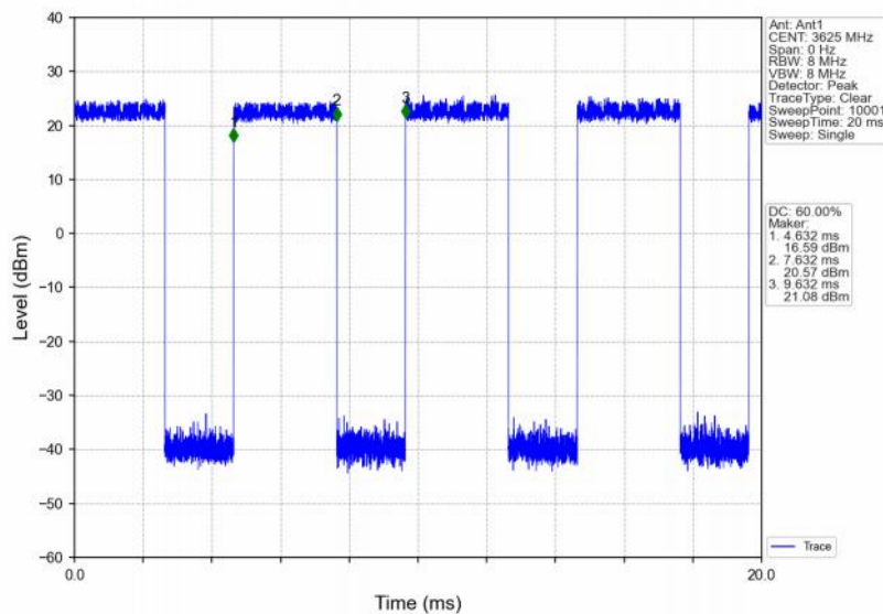
Band48_20MHz_QPSK_MCH_3625MHz_RB_50_25_NTNV
