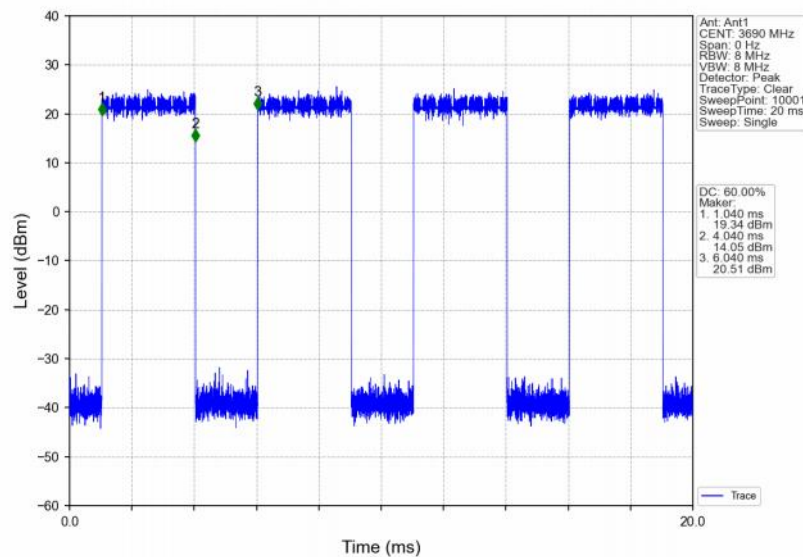
Band48_20MHz_16QAM_HCH_3690MHz_RB_100_0_NTNV
