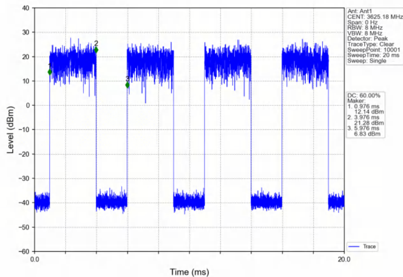
Band48_15MHz_256QAM_MCH_3625MHz_RB_1_38_NTNV
