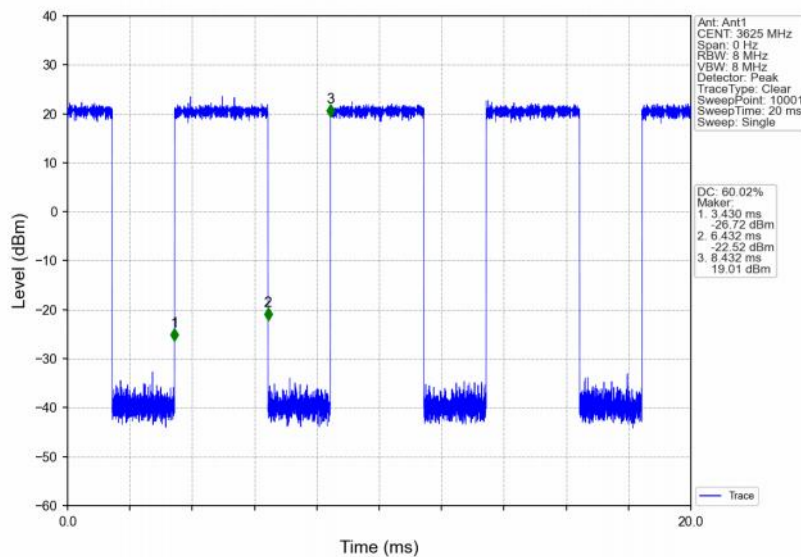
Band48_20MHz_QPSK_MCH_3625MHz_RB_100_0_NTNV
