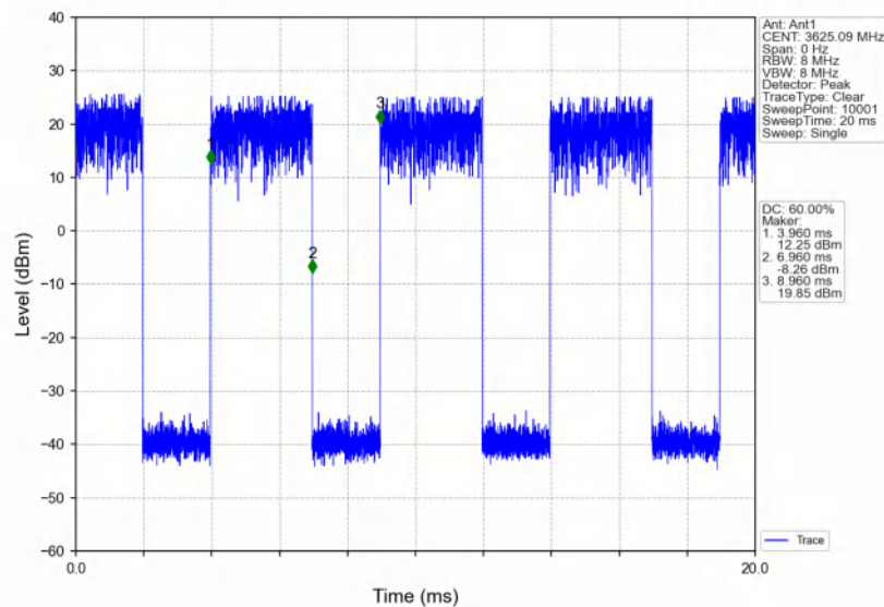
Band48_20MHz_16QAM_MCH_3625MHz_RB_1_50_NTNV
