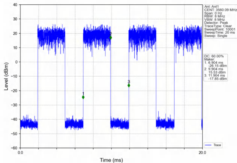
Band48_20MHz_64QAM_LCH_3560MHz_RB_1_50_NTNV
