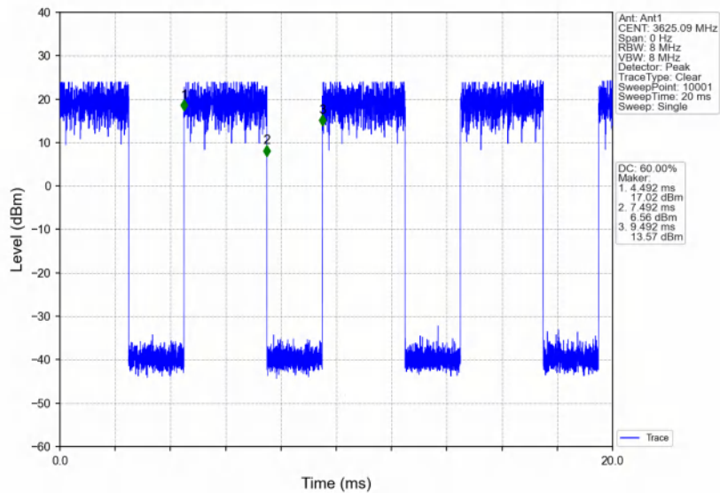
Band48_20MHz_QPSK_MCH_3625MHz_RB_1_99_NTNV
