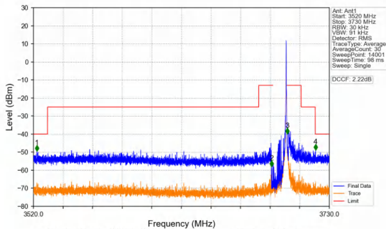
Band48_10MHz_QPSK_HCH_3695MHz_RB_1_49_NTNV
