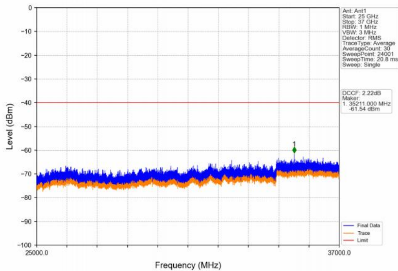
Band48_10MHz_QPSK_LCH_3555MHz_RB_1_0_NTNV
