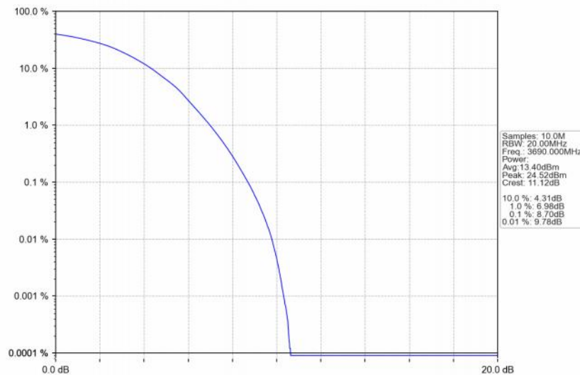
Band48_20MHz_16QAM_HCH_3690MHz_RB_100_0_NTNV
