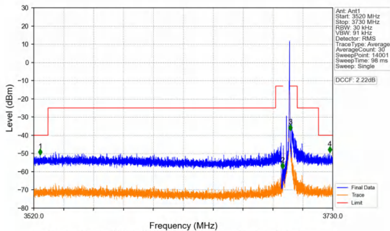
Band48_5MHz_QPSK_HCH_3697.5MHz_RB_1_24_NTNV
