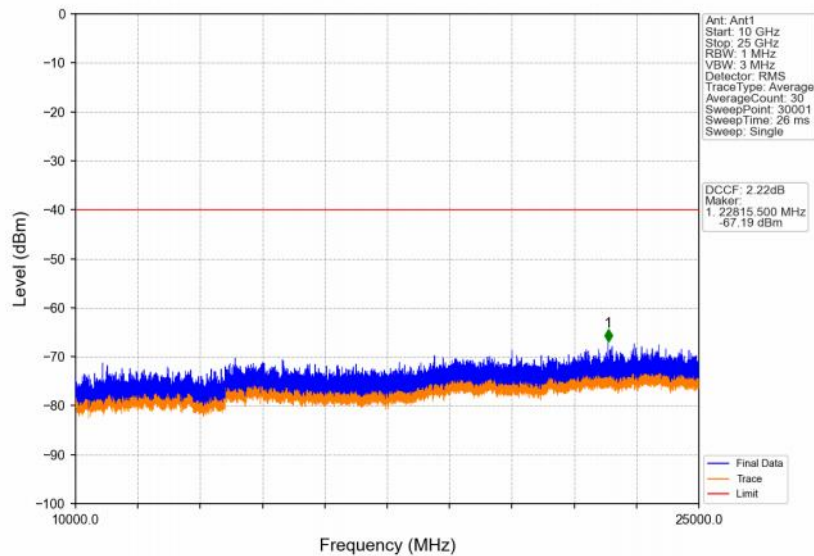
Band48_10MHz_QPSK_LCH_3555MHz_RB_1_0_NTNV
