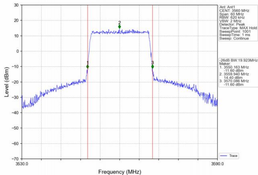
Band48_20MHz_256QAM_LCH_3560MHz_RB_100_0_NTNV
