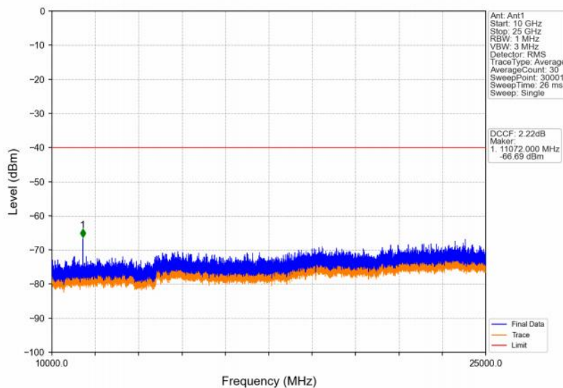
Band48_10MHz_QPSK_HCH_3695MHz_RB_1_0_NTNV
