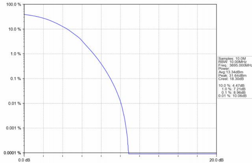
Band48_10MHz_QPSK_HCH_3695MHz_RB_50_0_NTNV
