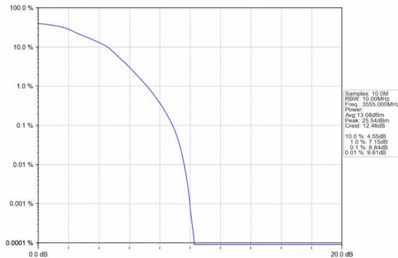
Band48_10MHz_16QAM_LCH_3555MHz_RB_50_0_NTNV
