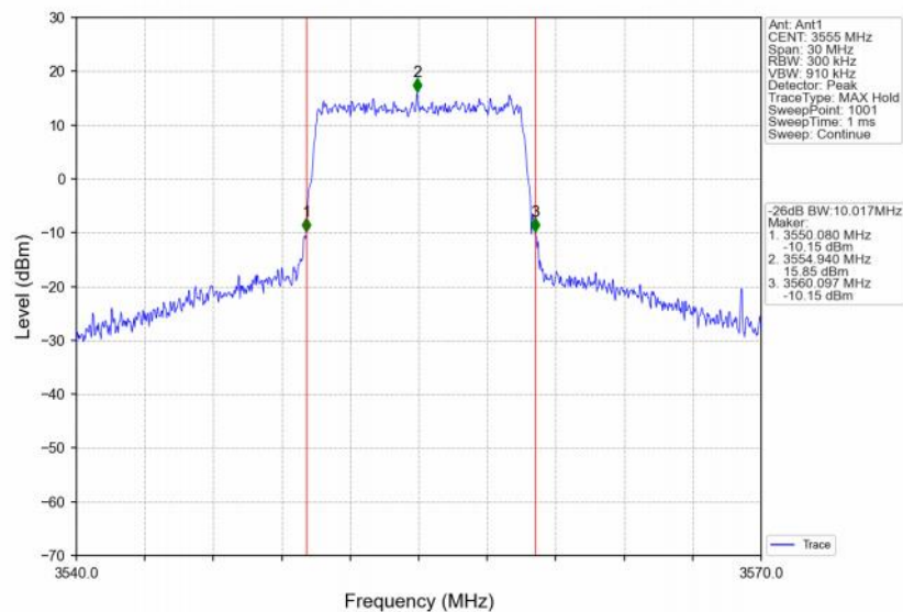
Band48_10MHz_16QAM_LCH_3555MHz_RB_50_0_NTNV
