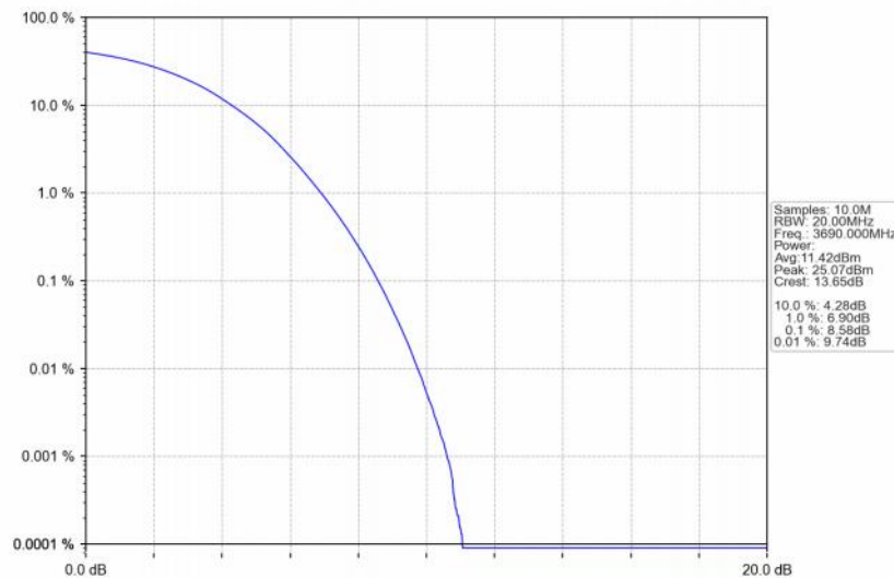
Band48_20MHz_256QAM_HCH_3690MHz_RB_100_0_NTNV
