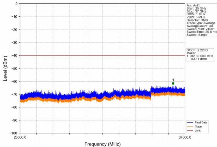
Band48_5MHz_QPSK_HCH_3697.5MHz_RB_1_24_NTNV
