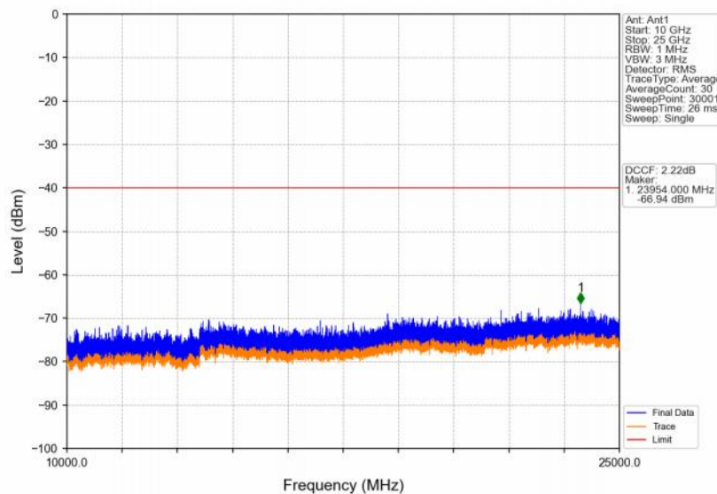
Band48_10MHz_16QAM_LCH_3555MHz_RB_1_0_NTNV
