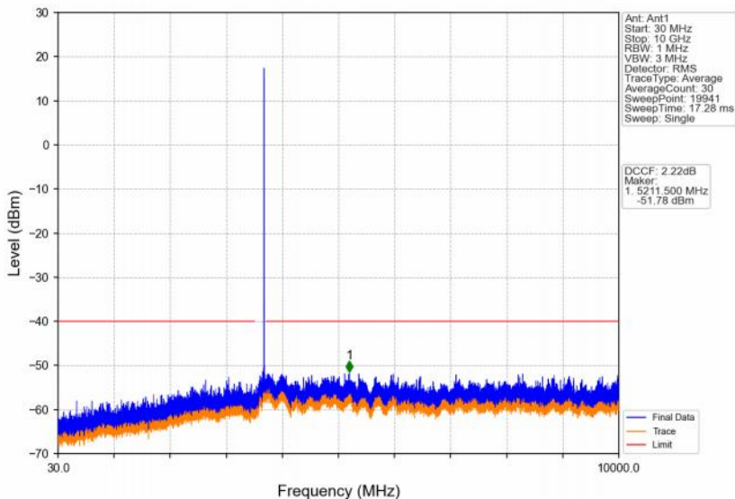
Band48_10MHz_QPSK_HCH_3695MHz_RB_1_0_NTNV
