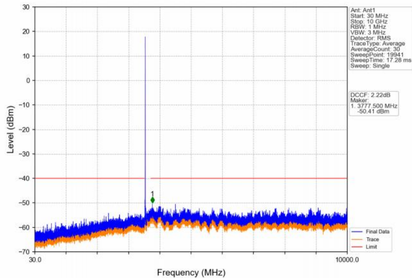
Band48_10MHz_16QAM_LCH_3555MHz_RB_1_0_NTNV
