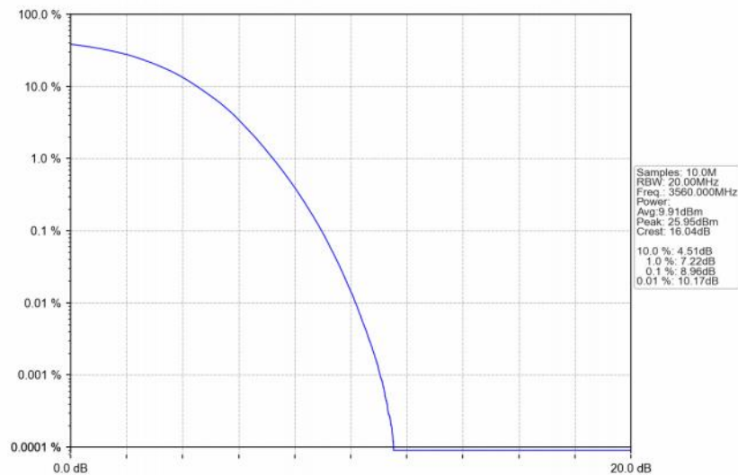
Band48_20MHz_256QAM_LCH_3560MHz_RB_100_0_NTNV
