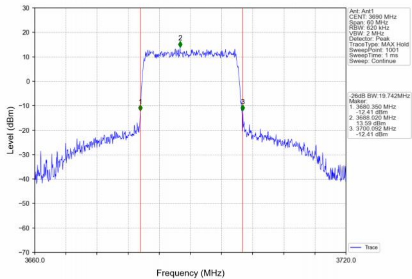
Band48_20MHz_256QAM_HCH_3690MHz_RB_100_0_NTNV
