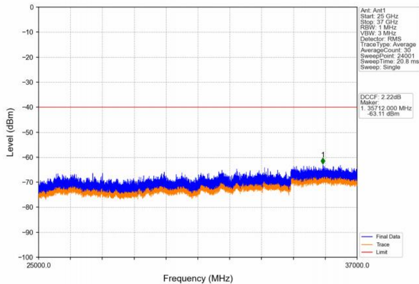
Band48_10MHz_QPSK_HCH_3695MHz_RB_1_49_NTNV
