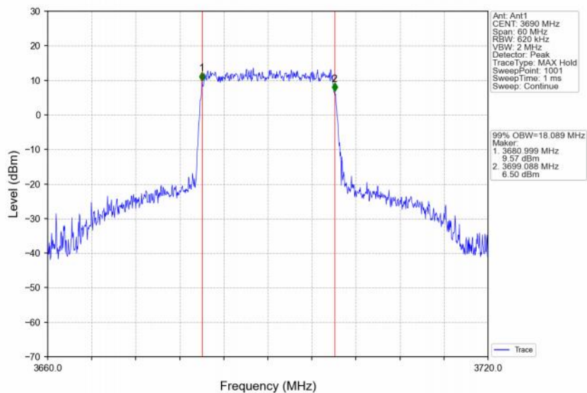
Band48_20MHz_256QAM_HCH_3690MHz_RB_100_0_NTNV
