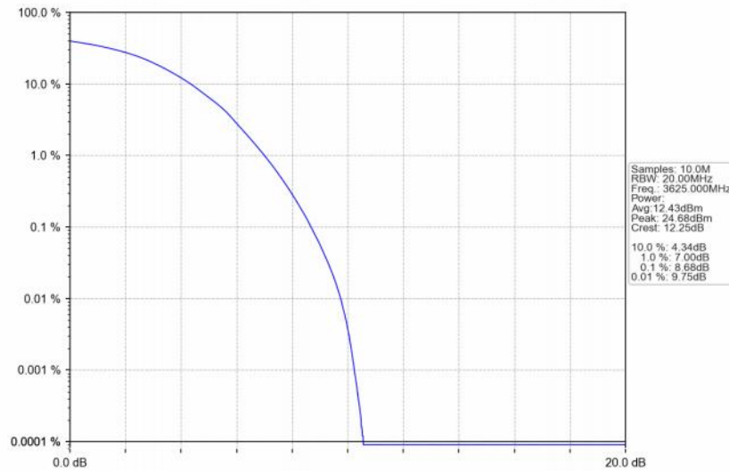
Band48_20MHz_16QAM_MCH_3625MHz_RB_100_0_NTNV
