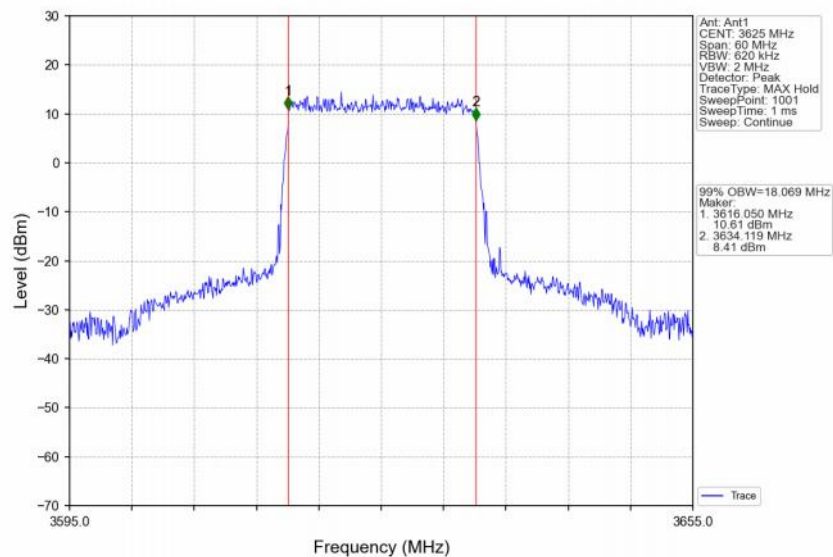
Band48_20MHz_QPSK_MCH_3625MHz_RB_100_0_NTNV
