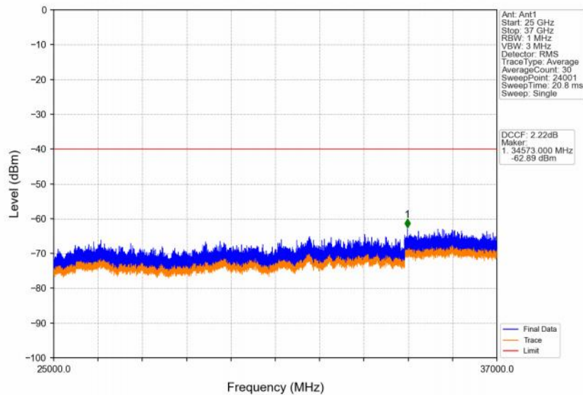
Band48_10MHz_16QAM_LCH_3555MHz_RB_50_0_NTNV
