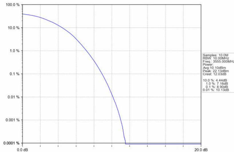
Band48_10MHz_256QAM_LCH_3555MHz_RB_50_0_NTNV
