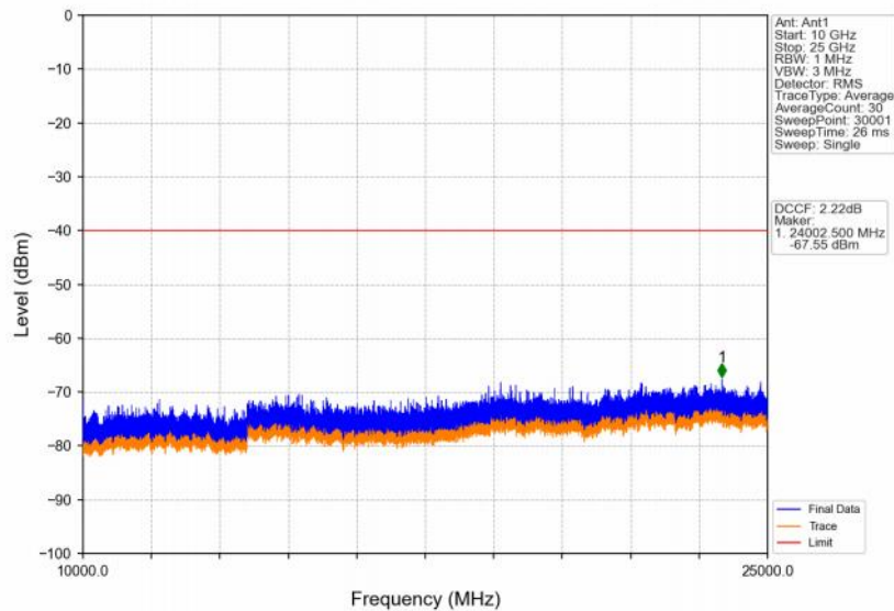
Band48_10MHz_QPSK_MCH_3625MHz_RB_1_0_NTNV
