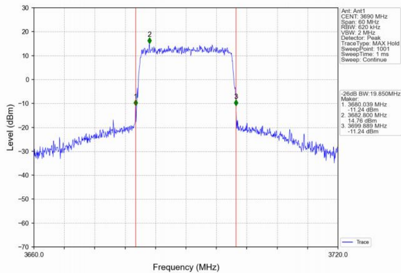
Band48_20MHz_16QAM_HCH_3690MHz_RB_100_0_NTNV
