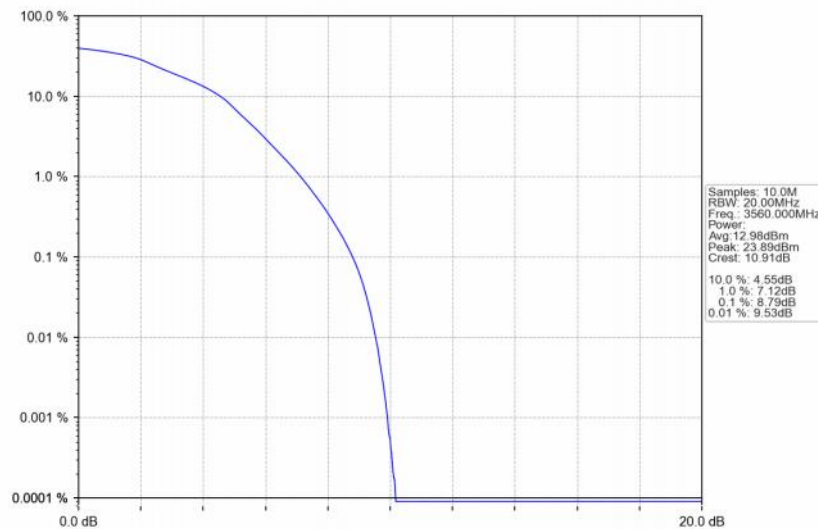
Band48_20MHz_16QAM_LCH_3560MHz_RB_100_0_NTNV
