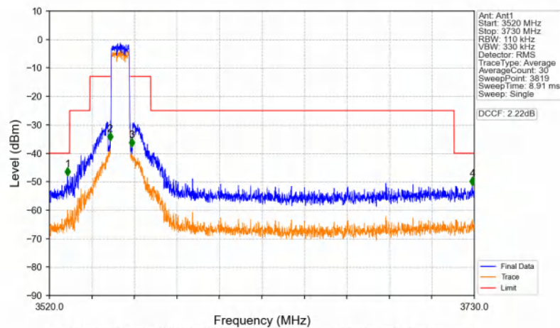
Band48_10MHz_16QAM_LCH_3555MHz_RB_50_0_NTNV
