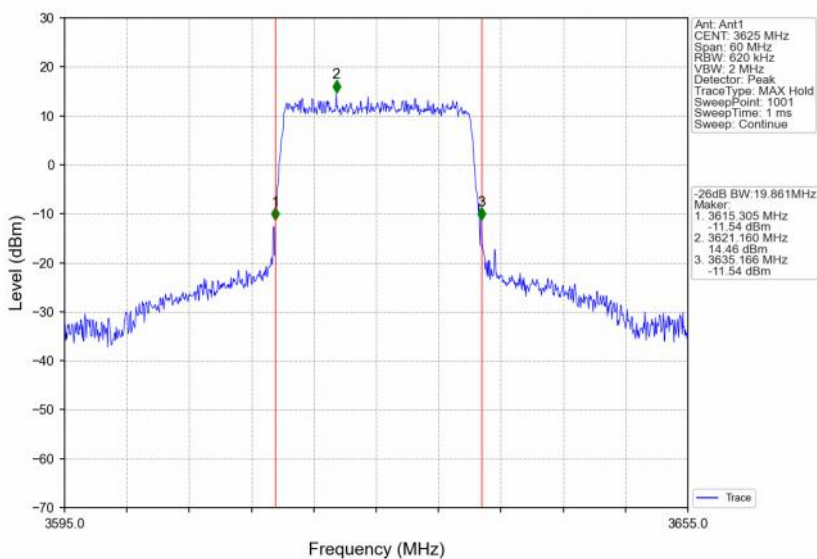
Band48_20MHz_QPSK_MCH_3625MHz_RB_100_0_NTNV
