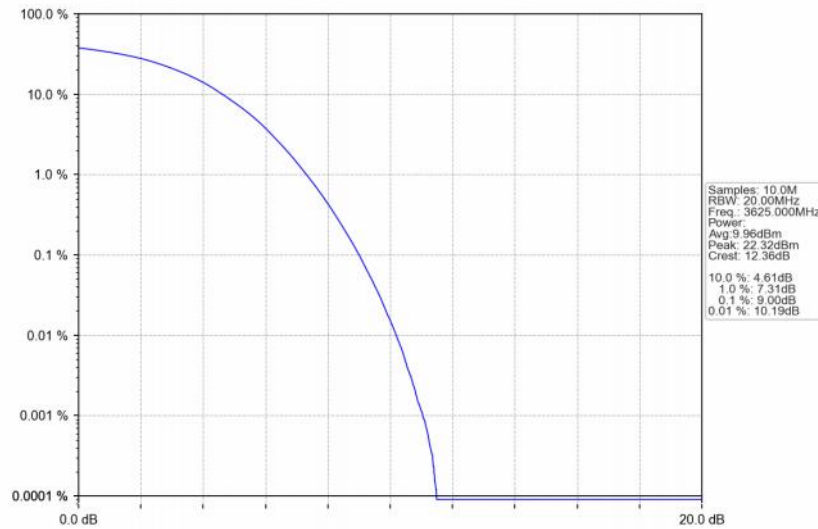
Band48_20MHz_256QAM_MCH_3625MHz_RB_100_0_NTNV
