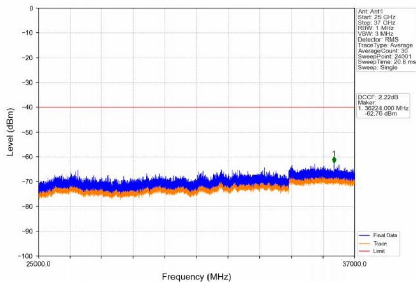
Band48_10MHz_QPSK_MCH_3625MHz_RB_1_0_NTNV
