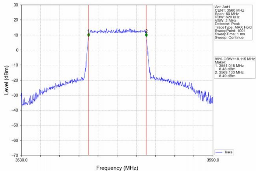
Band48_20MHz_256QAM_LCH_3560MHz_RB_100_0_NTNV
