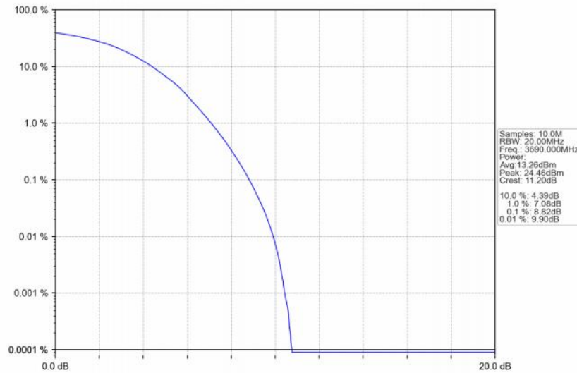
Band48_20MHz_QPSK_HCH_3690MHz_RB_100_0_NTNV
