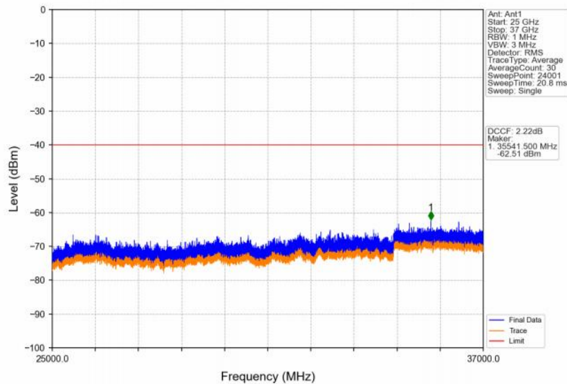
Band48_20MHz_256QAM_HCH_3690MHz_RB_1_0_NTNV
