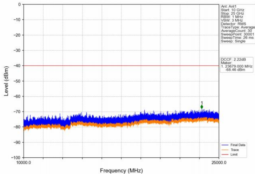
Band48_20MHz_QPSK_LCH_3560MHz_RB_1_0_NTNV
