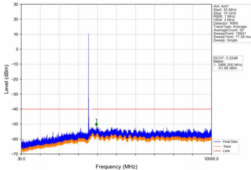
Band48_20MHz_256QAM_LCH_3560MHz_RB_1_0_NTNV
