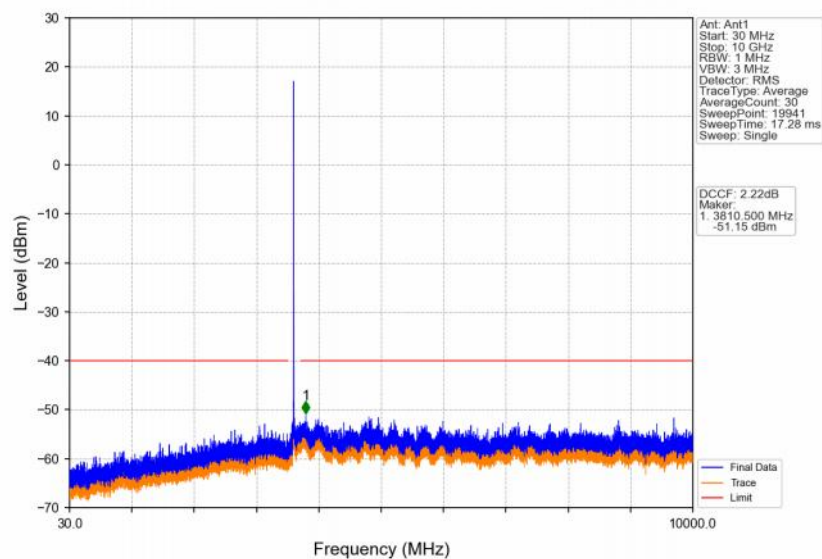
Band48_20MHz_QPSK_MCH_3625MHz_RB_1_0_NTNV
