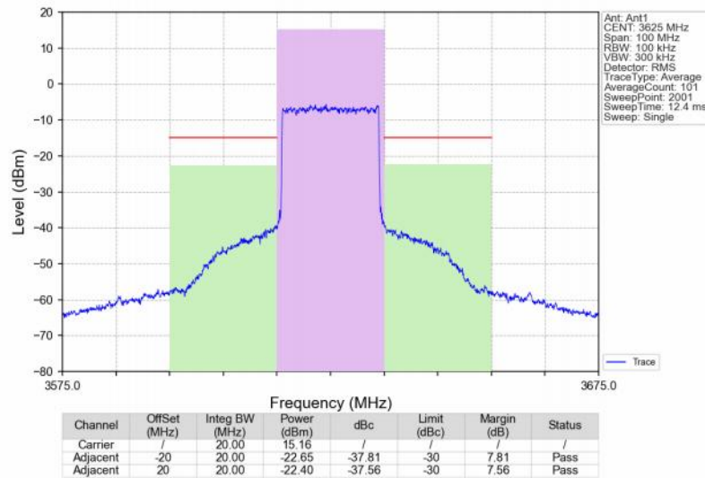
Band48_20MHz_256QAM_MCH_3625MHz_RB_100_0_NTNV
