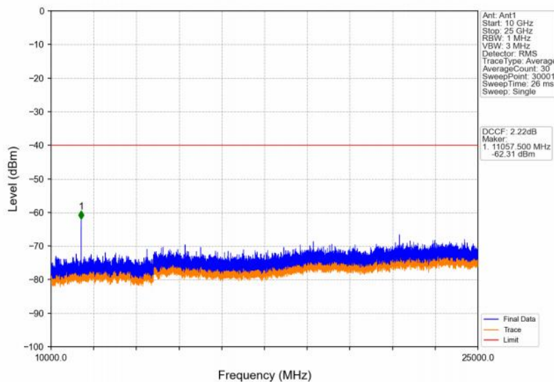
Band48_15MHz_QPSK_HCH_3692.5MHz_RB_1_0_NTNV
