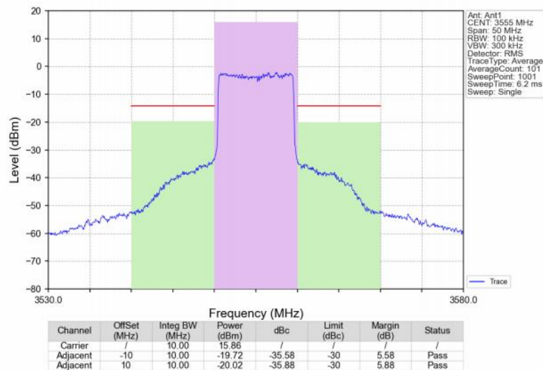
Band48 10MHz 256QAM LCH 3555MHz RB 50 0 NTN
