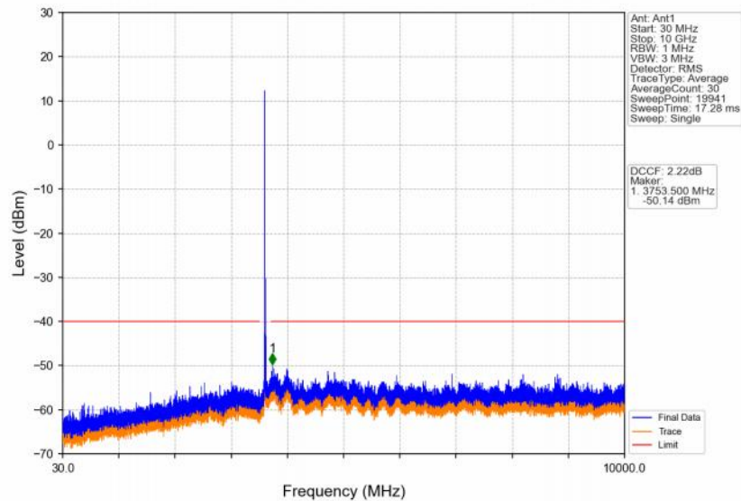
Band48_20MHz_256QAM_MCH_3625MHz_RB_1_0_NTNV
