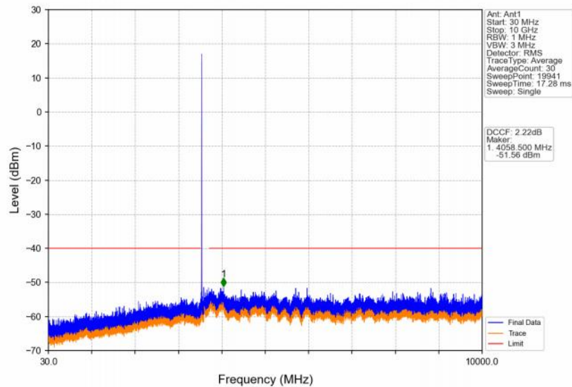
Band48_20MHz_16QAM_LCH_3560MHz_RB_1_0_NTNV
