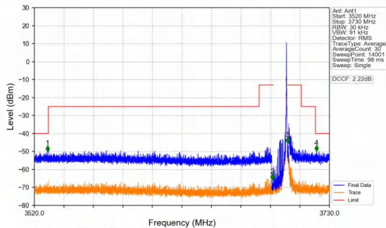
Band48_10MHz_64QAM_HCH_3695MHz_RB_1_49_NTNV
