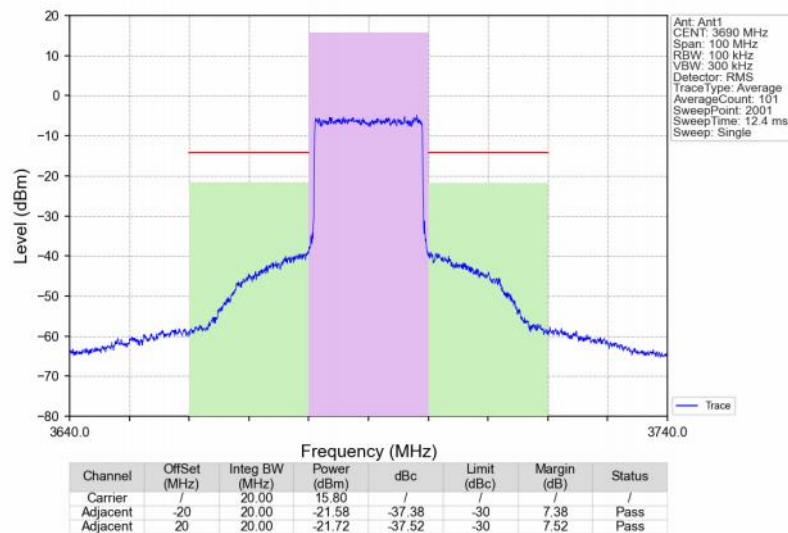
Band48_20MHz_256QAM_HCH_3690MHz_RB_100_0_NTNV
