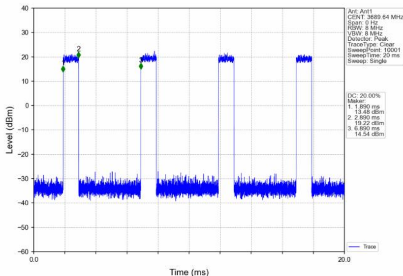
n48_30kHz_SISO_NTNV_20MHz_DFT-s-OFDM QPSK_3690MHz_Inner_Full
