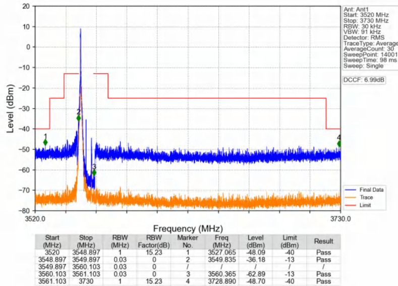
n48_30kHz_SISO_NTNV_10MHz_DFT-s-OFDM QPSK_3555MHz_Inner_1RB_Left
