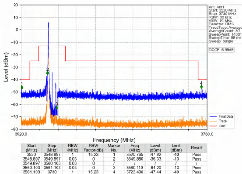
n48_30kHz_SISO_NTNV_10MHz_DFT-s-OFDM QPSK 3555MHz_Edge_1RB_Left
