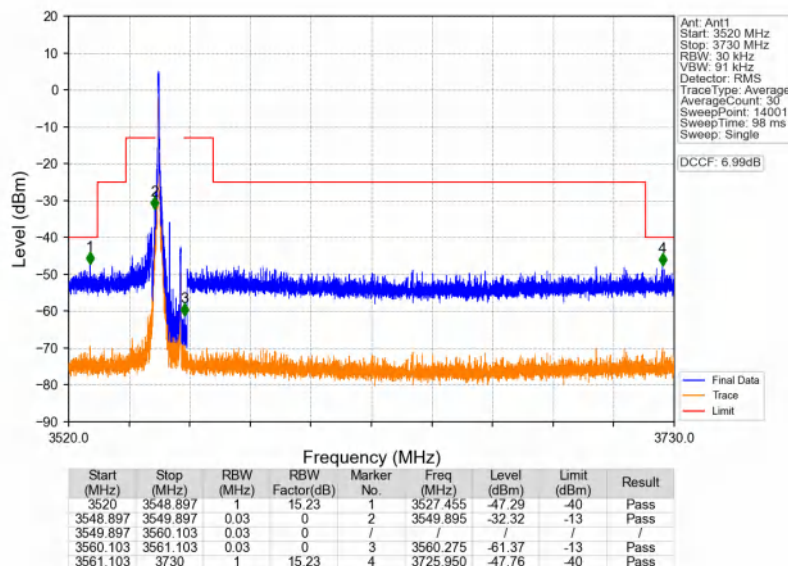
n48_30kHz_SISO_NTNV_10MHz_CP-OFDM_QPSK_3555MHz_Inner_1RB_Left
