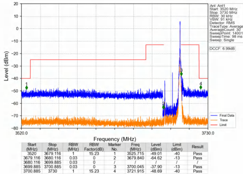
n48_30kHz_SISO_NTNV_20MHz_CP-OFDM QPSK_3690MHz_Inner_1RB_Right
