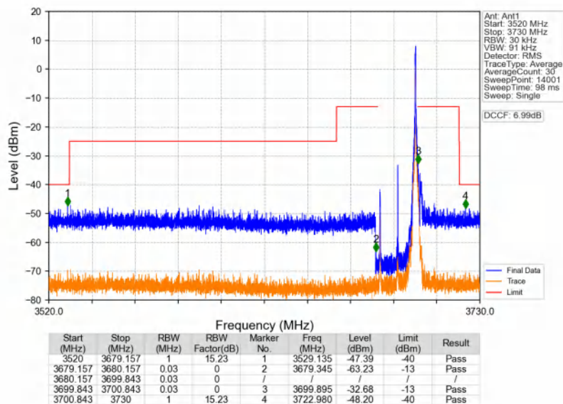
n48_30kHz_SISO_NTNV_20MHz_DFT-s-OFDM QPSK_3690MHz_Inner_1RB_Right
