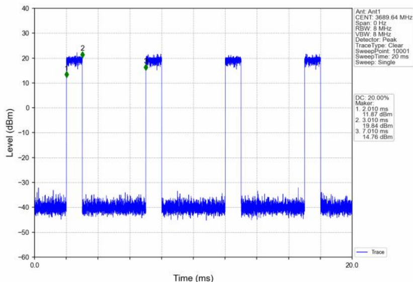
n48_30kHz_SISO_NTNV_20MHz_CP-OFDM QPSK_3690MHz_Inner_Full
