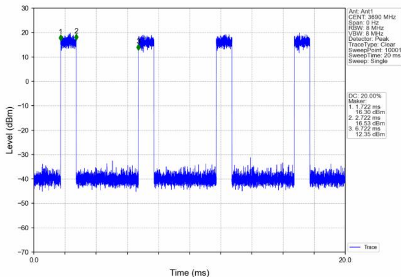
n48_30kHz_SISO_NTNV_20MHz_CP-OFDM QPSK_3690MHz_Inner_Full
