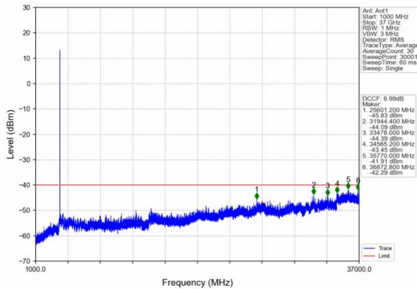
n48_30kHz_SISO_NTNV_10MHz_DFT-s-OFDM QPSK_3555MHz_Edge_1RB_Left
