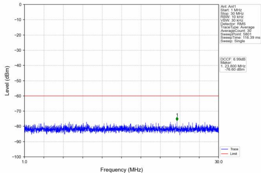
n48_30kHz_SISO_NTNV_10MHz_DFT-s-OFDM QPSK_3555MHz_Edge_1RB_Left
