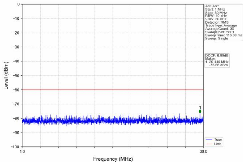
n48_30kHz_SISO_NTNV_10MHz_DFT-s-OFDM QPSK_3555MHz_Inner_1RB_Left
