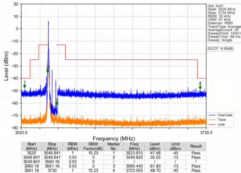
n48_30kHz_SISO_NTNV_10MHz_DFT-s-OFDM PI/2 BPSK_3555MHz_Edge_1RB_Left
