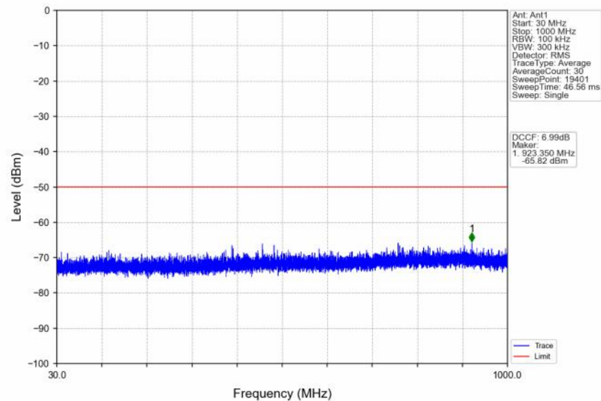
n48_30kHz_SISO_NTNV_10MHz_DFT-s-OFDM QPSK_3555MHz_Edge_1RB_Left
