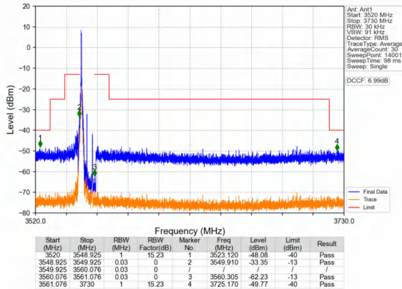
n48_30kHz_SISO_NTNV_10MHz_DFT-s-OFDM PI/2 BPSK_3555MHz_Inner_1RB_Left
