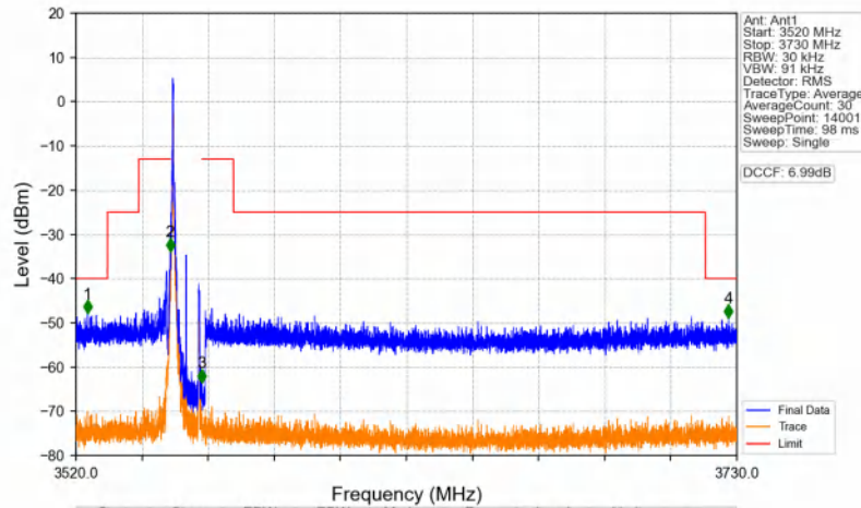
n48_30kHz_SISO_NTNV_10MHz_DFT-s-OFDM QPSK_3555MHz_Edge_1RB_Left
