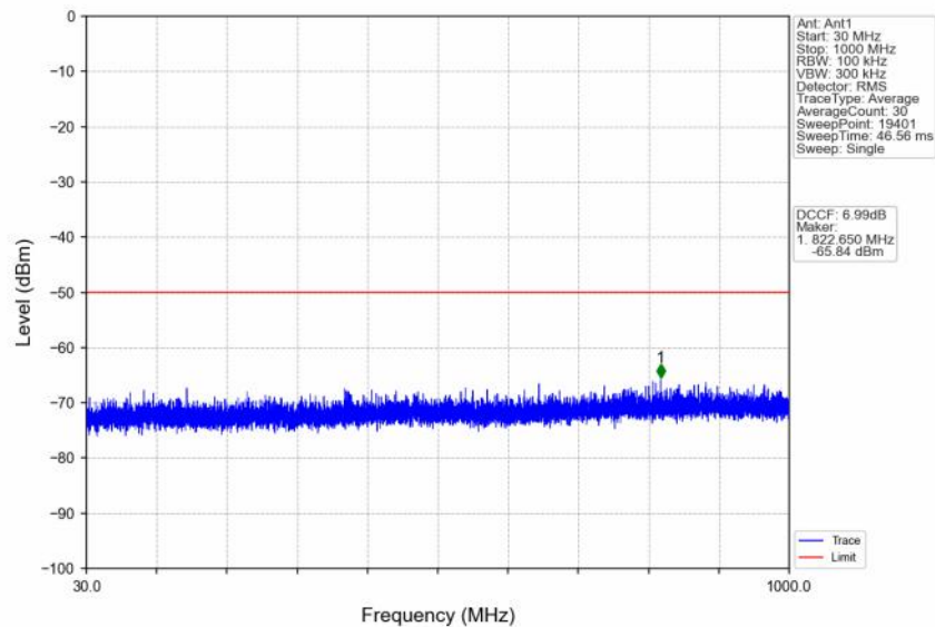
n48_30kHz_SISO_NTNV_10MHz_DFT-s-OFDM QPSK_3555MHz_Inner_1RB_Left
