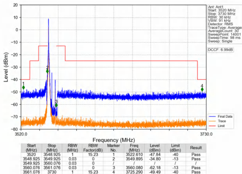
n48_30kHz_SISO_NTNV_10MHz_DFT-s-OFDM QPSK_3555MHz_Inner_1RB_Left
