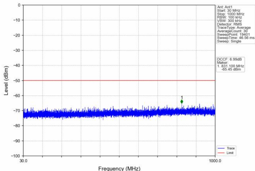
n48_30kHz_SISO_NTNV_10MHz_DFT-s-OFDM PI/2 BPSK_3555MHz_Edge_1RB_Left
