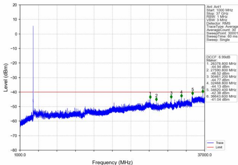
n48_30kHz_SISO_NTNV_10MHz_DFT-s-OFDM QPSK_3555MHz_Inner_1RB_Left
