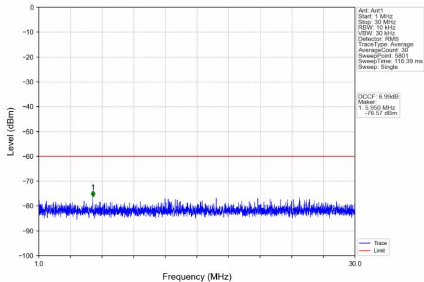
n48_30kHz_SISO_NTNV_10MHz_CP-OFDM_QPSK_3555MHz_Inner_1RB_Left
