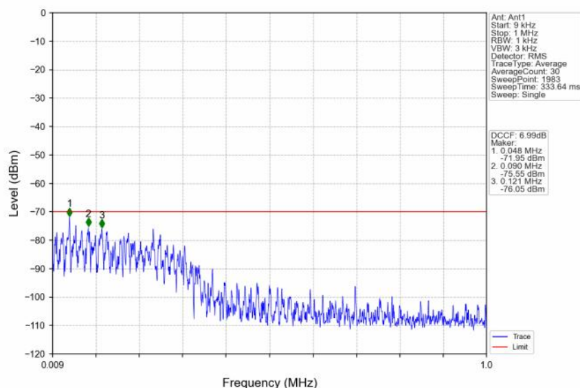
n48_30kHz_SISO_NTNV_10MHz_CP-OFDM_QPSK_3555MHz_Inner_1RB_Left
