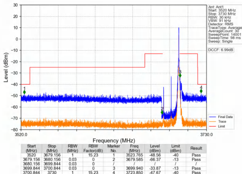
n48_30kHz_SISO_NTNV_20MHz_DFT-s-OFDM PI/2 BPSK_3690MHz_Inner_1RB_Right
