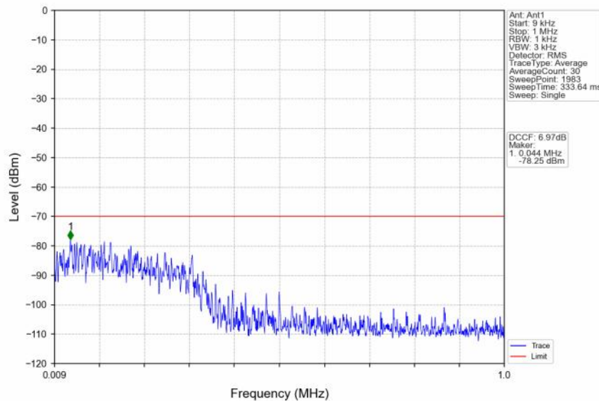
n48_30kHz_SISO_NTNV_10MHz_CP-OFDM_QPSK_3555MHz_Edge_1RB_Left
