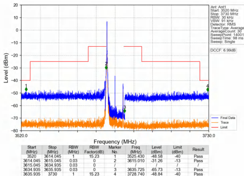
n48_30kHz_SISO_NTNV_20MHz_CP-OFDM QPSK_3624.99MHz_Edge_1RB_Left
