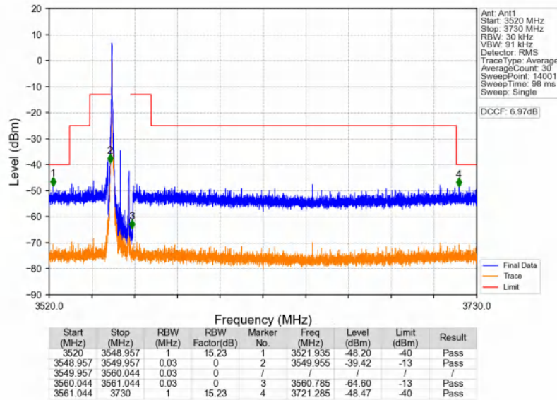
n48_30kHz_SISO_NTNV_10MHz_CP-OFDM_QPSK_3555MHz_Edge_1RB_Left
