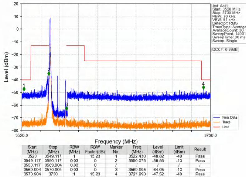
n48_30kHz_SISO_NTNV_20MHz_DFT-s-OFDM QPSK_3560.01MHz_Inner_1RB_Left
