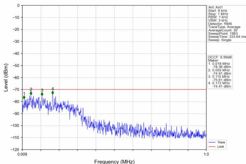
n48_30kHz_SISO_NTNV_20MHz_CP-OFDM_QPSK_3560.01MHz_Inner_1RB_Left
