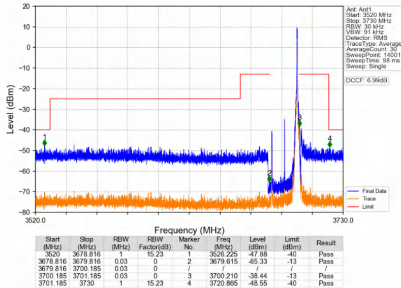
n48_30kHz_SISO_NTNV_20MHz_DFT-s-OFDM QPSK_3690MHz_Inner_1RB_Right
