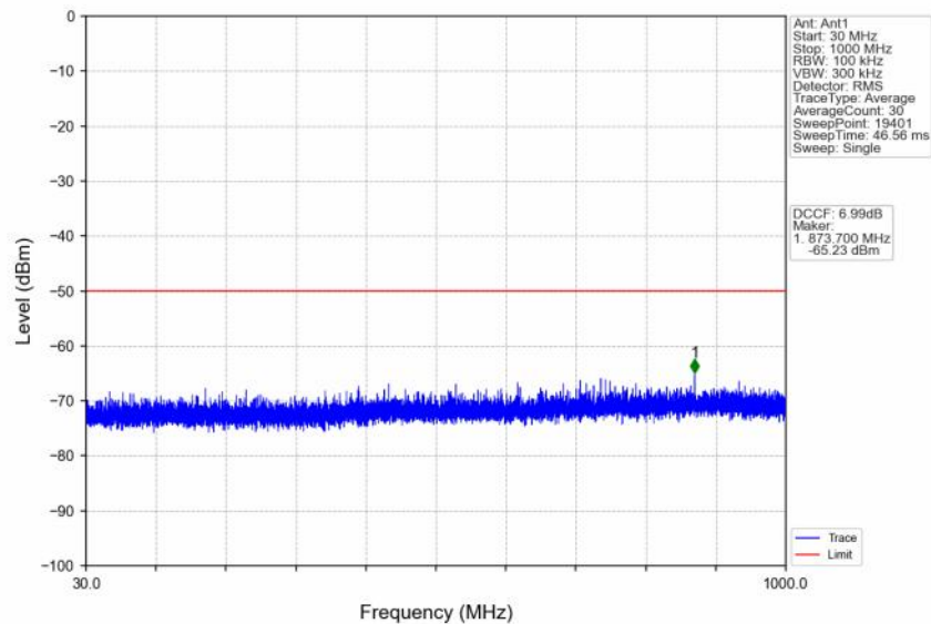
n48_30kHz_SISO_NTNV_10MHz_CP-OFDM_QPSK_3555MHz_Inner_1RB_Left
