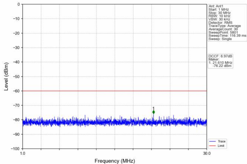
n48_30kHz_SISO_NTNV_10MHz_CP-OFDM_QPSK_3555MHz_Edge_1RB_Left
