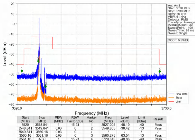
n48_30kHz_SISO_NTNV_10MHz_CP-OFDM_QPSK_3555MHz_Inner_1RB_Left
