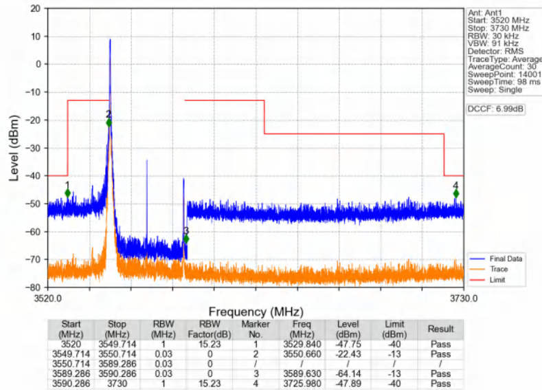
n48_30kHz_SISO_NTNV_40MHz_DFT-s-OFDM QPSK_3570MHz_Inner_1RB_Left
