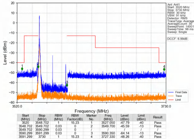
n48_30kHz_SISO_NTNV_40MHz_CP-OFDM_QPSK_3570MHz_Inner_1RB_Left
