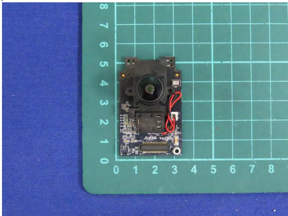
(50) EUT Photo
