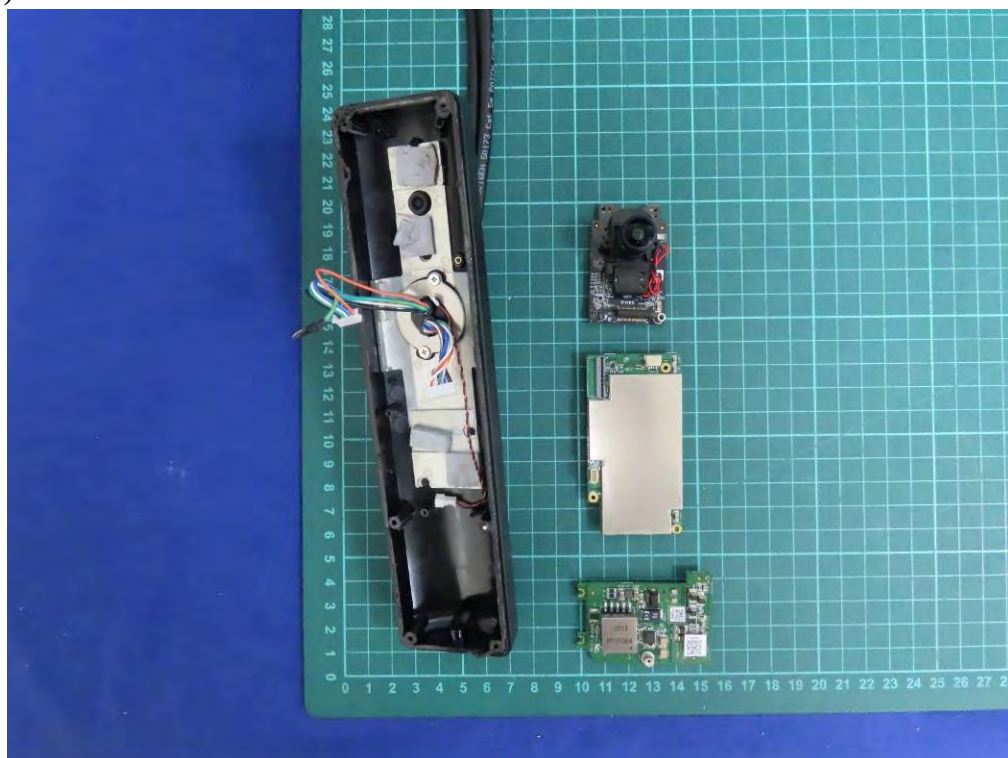
(49) EUT Photo
