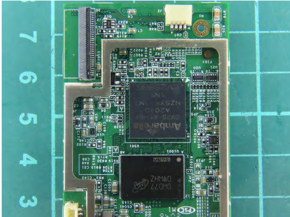
(57) EUT Photo
