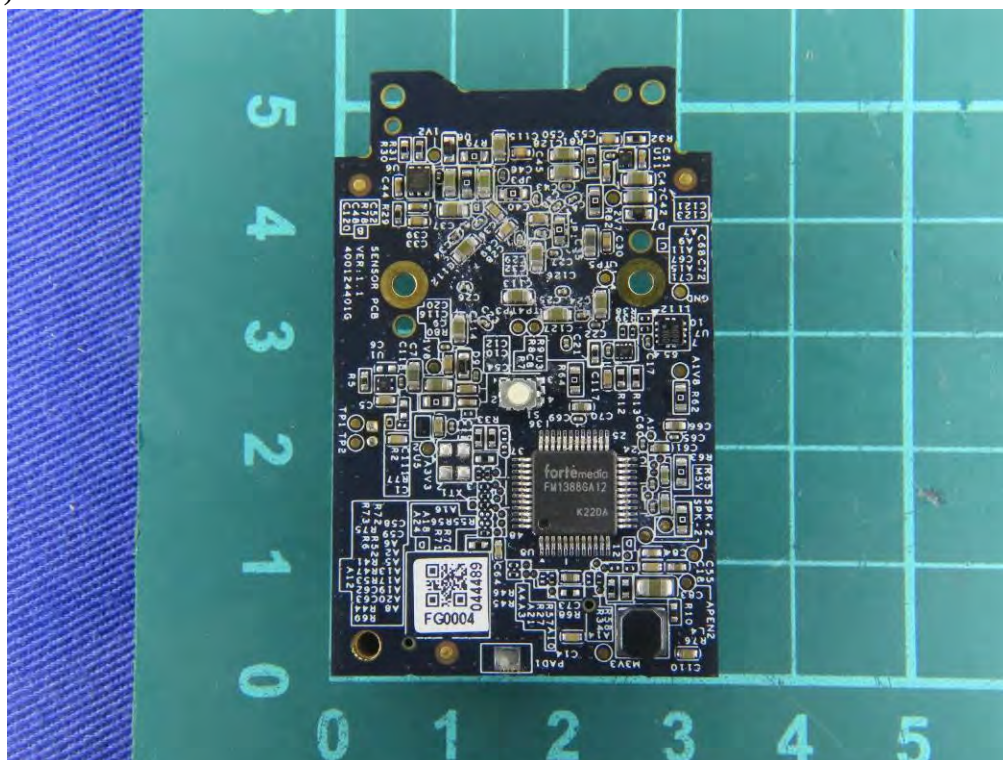
(53) EUT Photo
