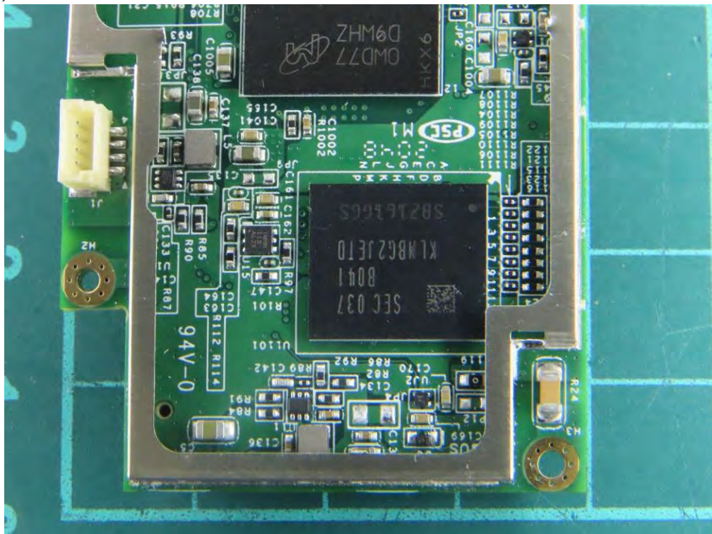
(58) EUT Photo
