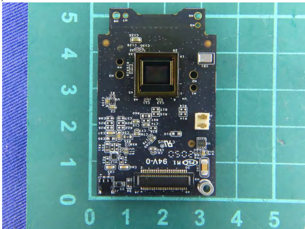
(52) EUT Photo
