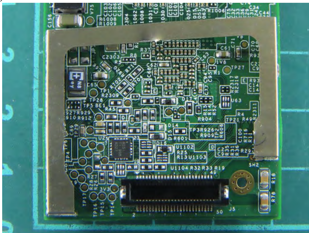
(63) EUT Photo
