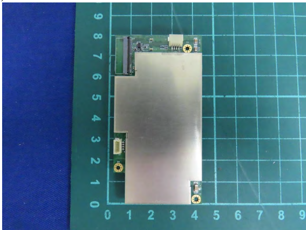
(54) EUT Photo
