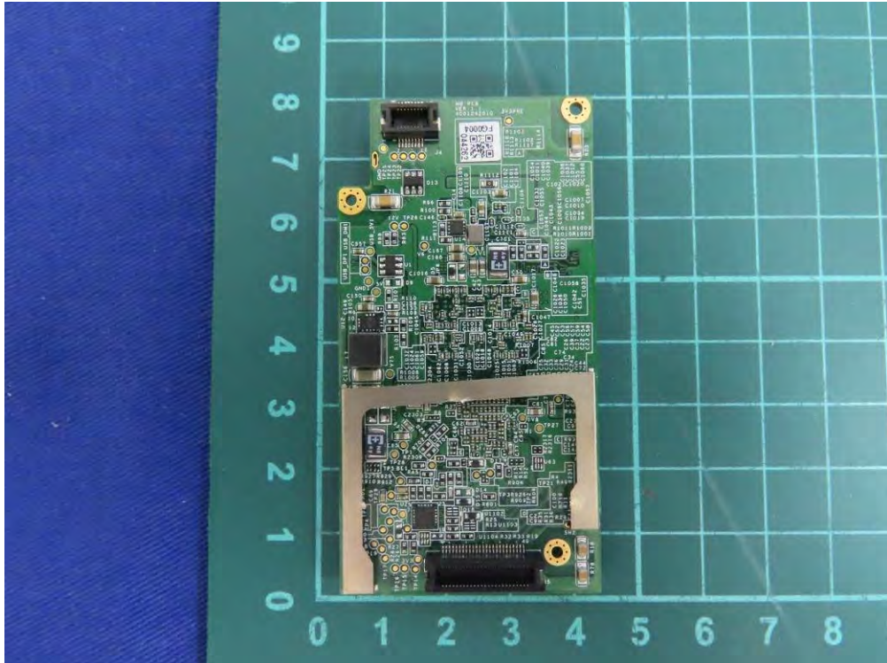
(61) EUT Photo
