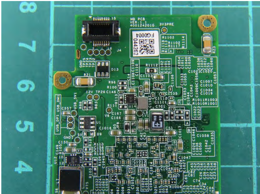
(62) EUT Photo
