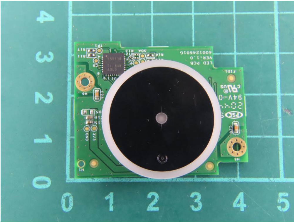
(12) EUT Photo
