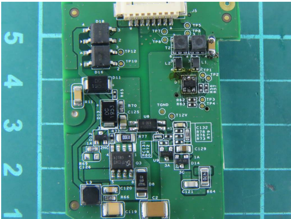
(52) EUT Photo
