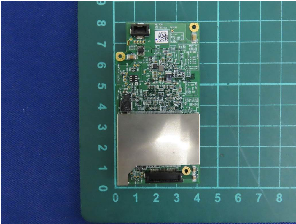
(44) EUT Photo
