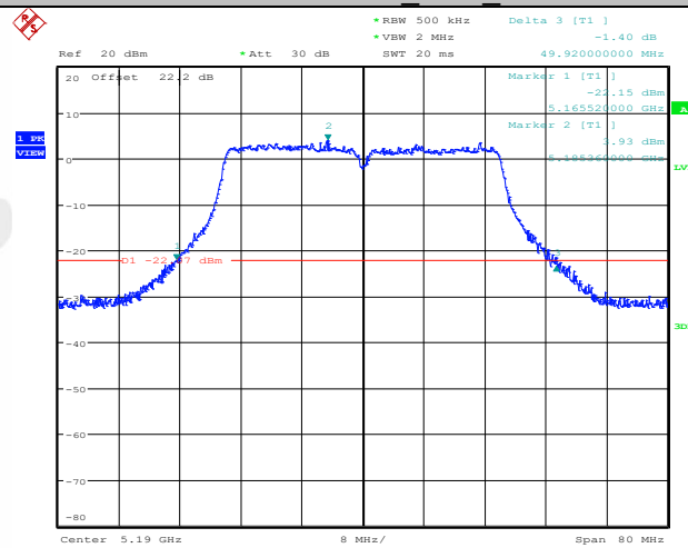
11N40SISO Ant1 5190
