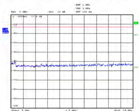
LTE Band 66 20MHz CH-Middle 3GHz~18GHz
