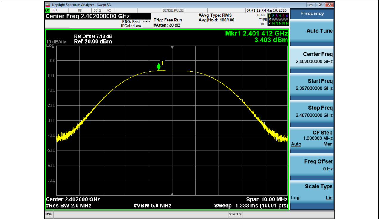
Peak Power NVNT BLE 2M 2402MHz Ant1
