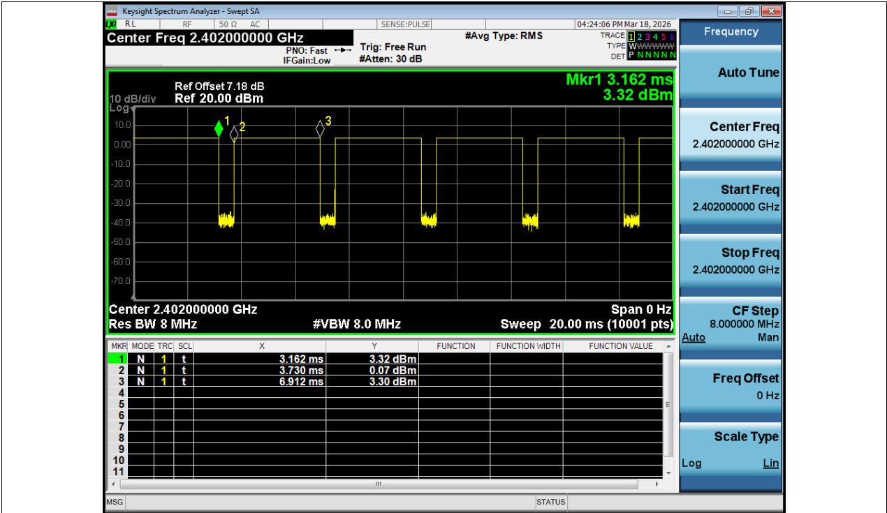
Duty Cycle NVNT BLE 1M 2402MHz Ant1
