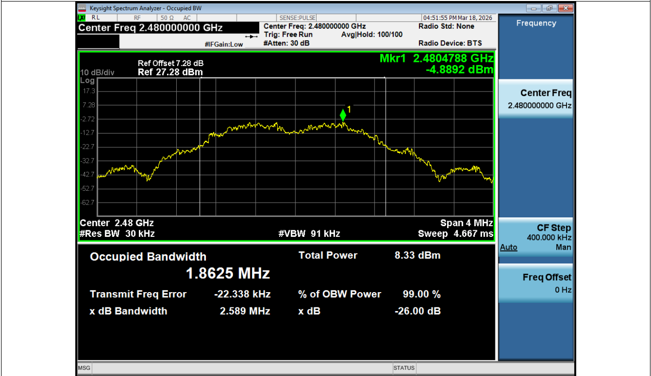
OBW NVNT BLE 2M 2480MHz Ant1
