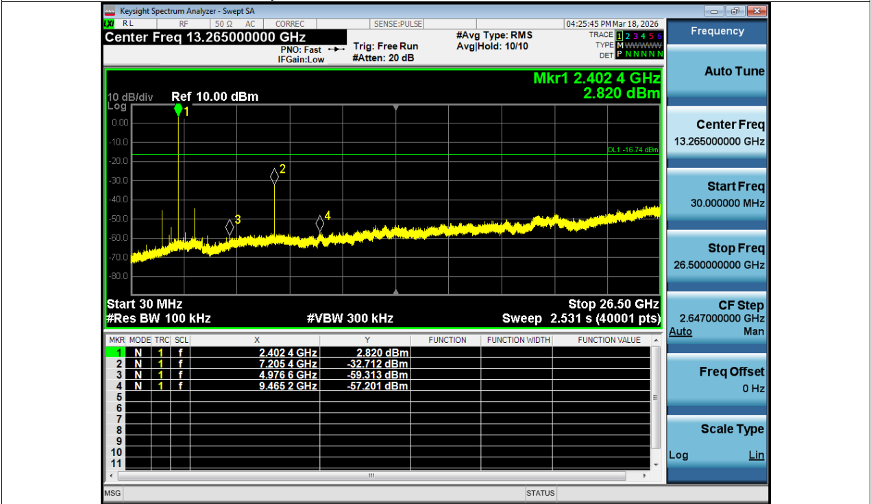
Tx. Spurious NVNT BLE 1M 2402MHz Ant1 Emission
