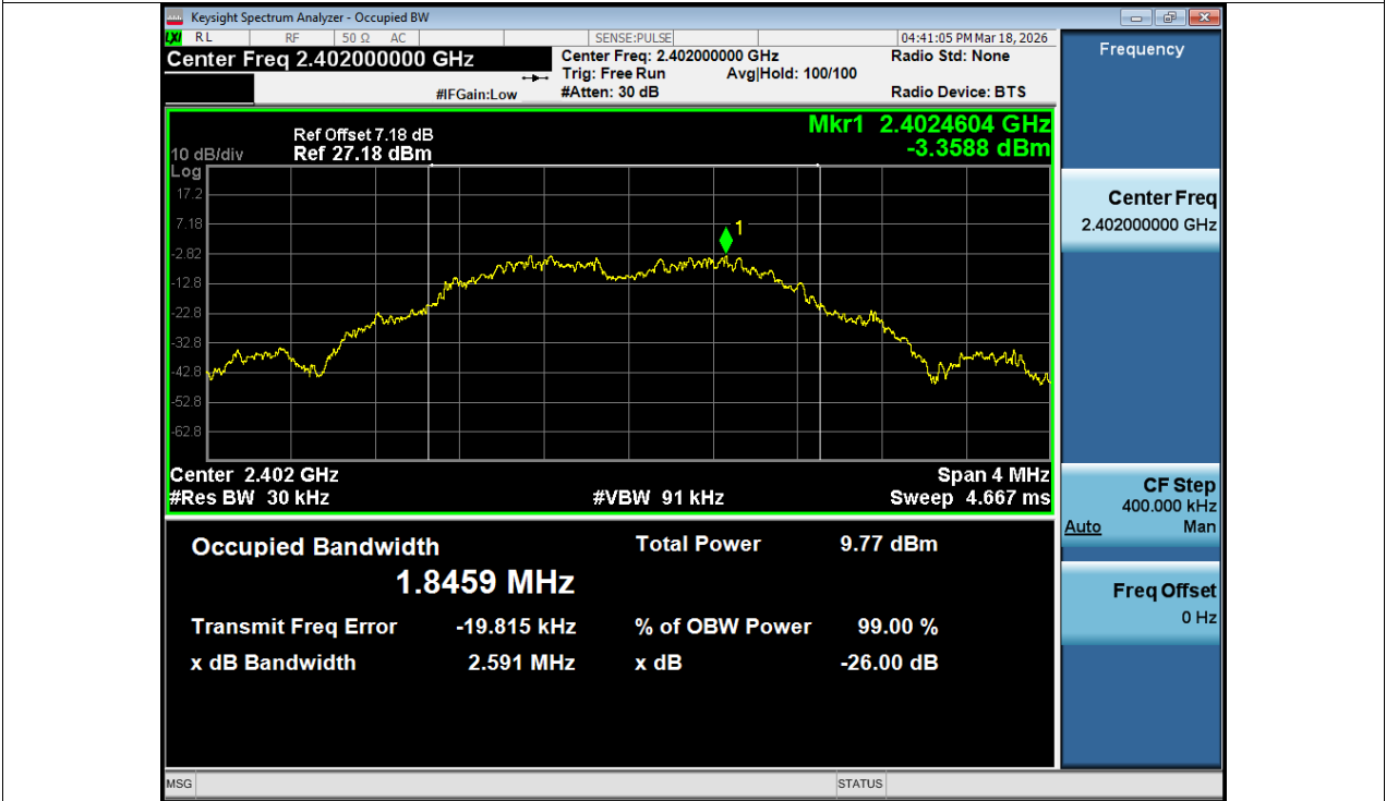
OBW NVNT BLE 2M 2402MHz Ant1
