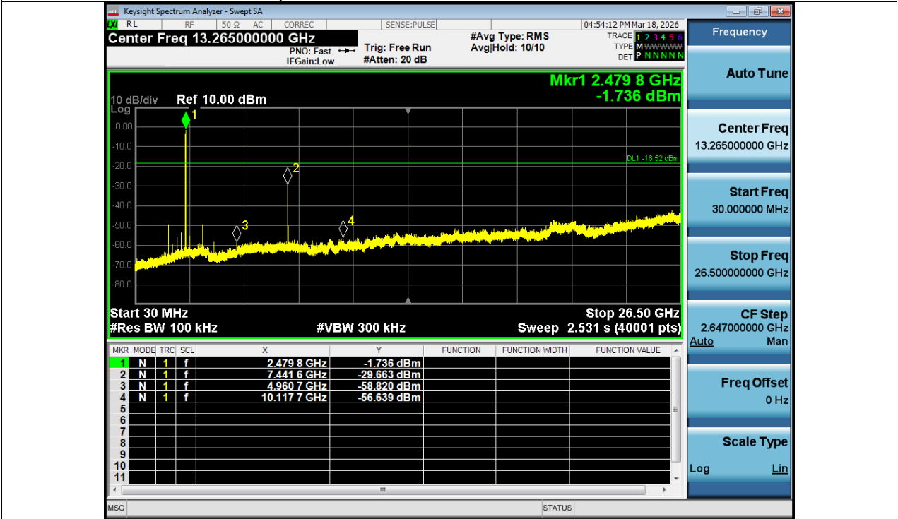
Tx. Spurious NVNT BLE 2M 2480MHz Ant1 Emission
