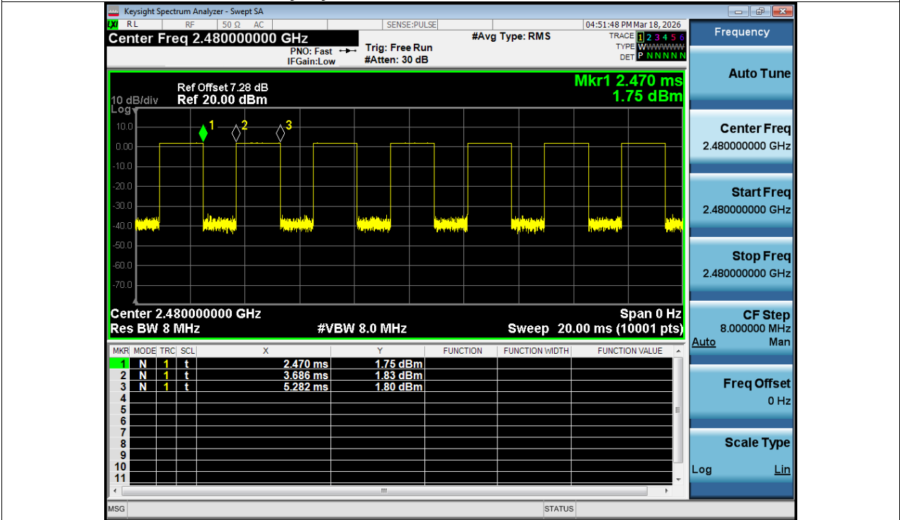
Duty Cycle NVNT BLE 2M 2480MHz Ant1
