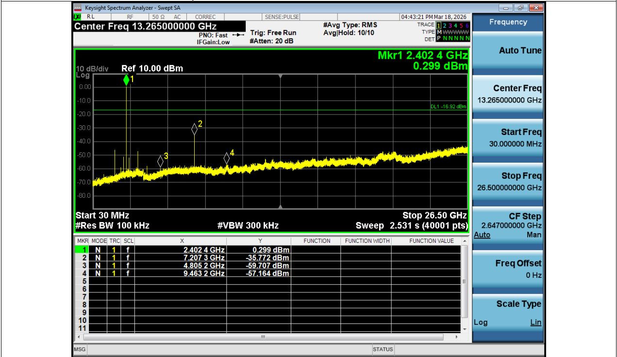
Tx. Spurious NVNT BLE 2M 2402MHz Ant1 Emission
