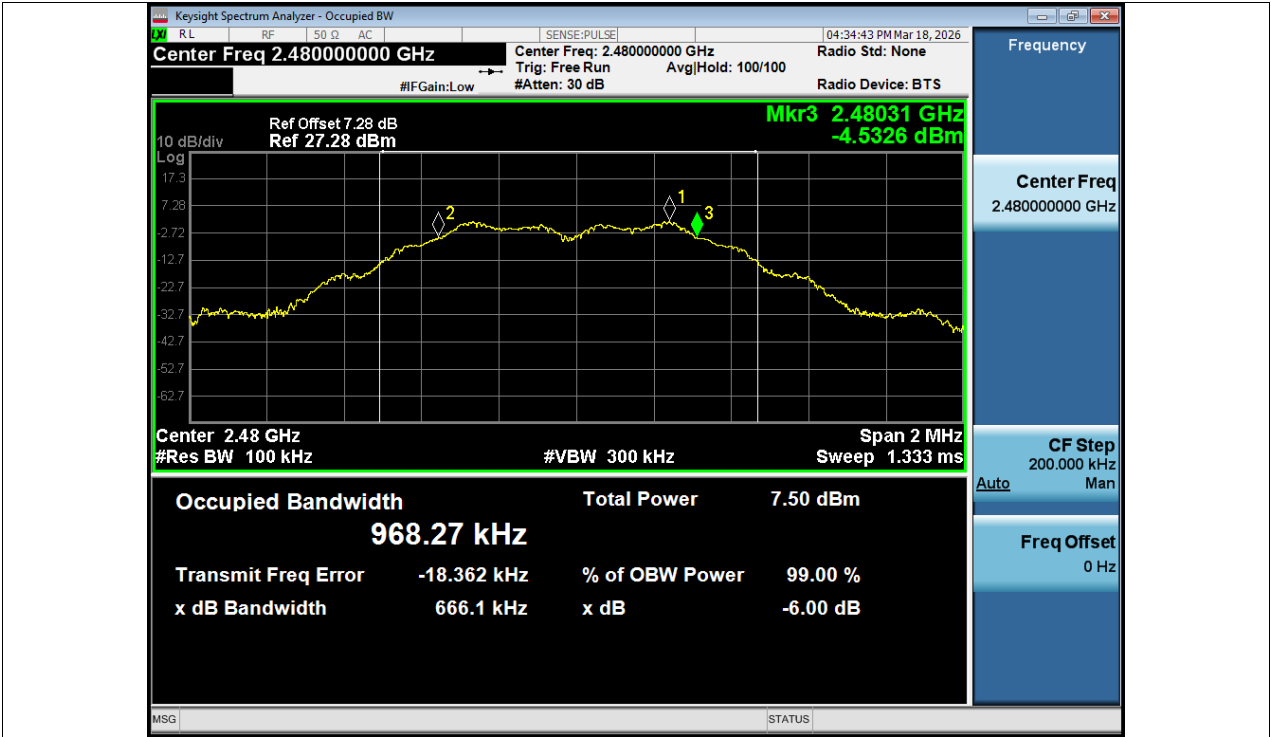
-6dB Bandwidth NVNT BLE 1M 2480MHz Ant1
