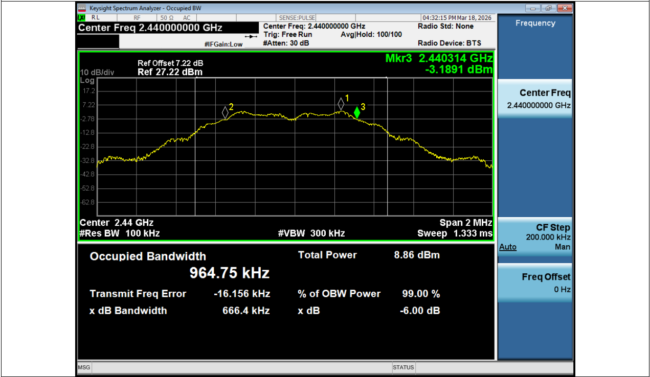
-6dB Bandwidth NVNT BLE 1M 2440MHz Ant1
