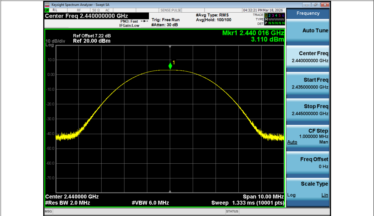
Peak Power NVNT BLE 1M 2440MHz Ant1
