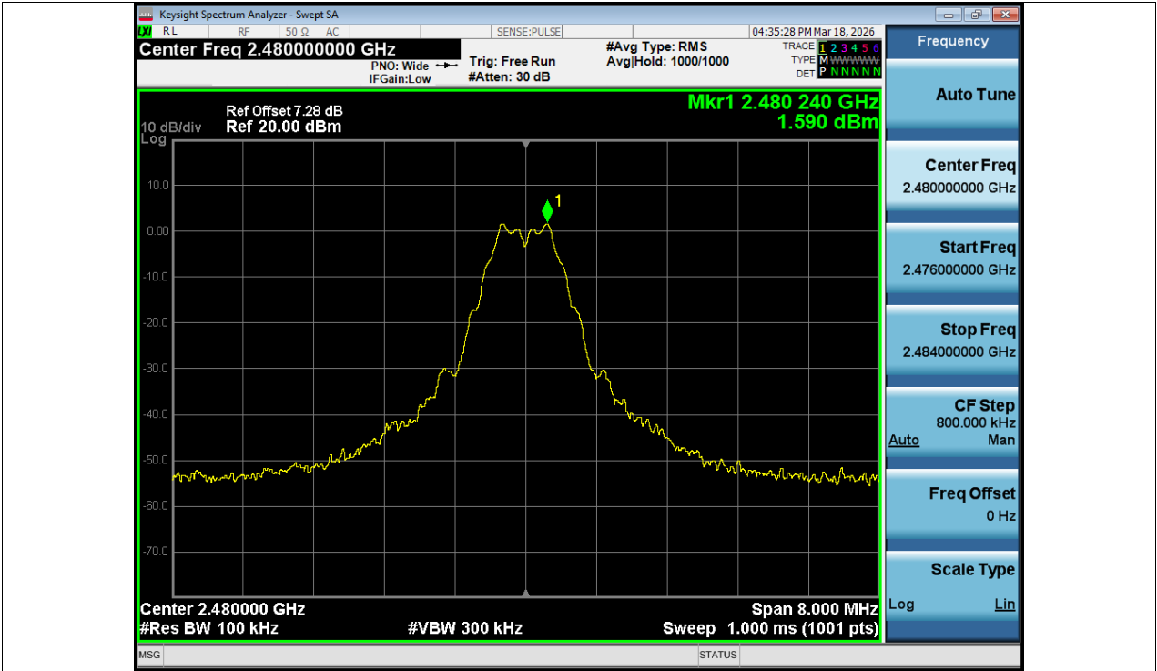
Band Edge NVNT BLE 1M 2480MHz Ant1 Ref
