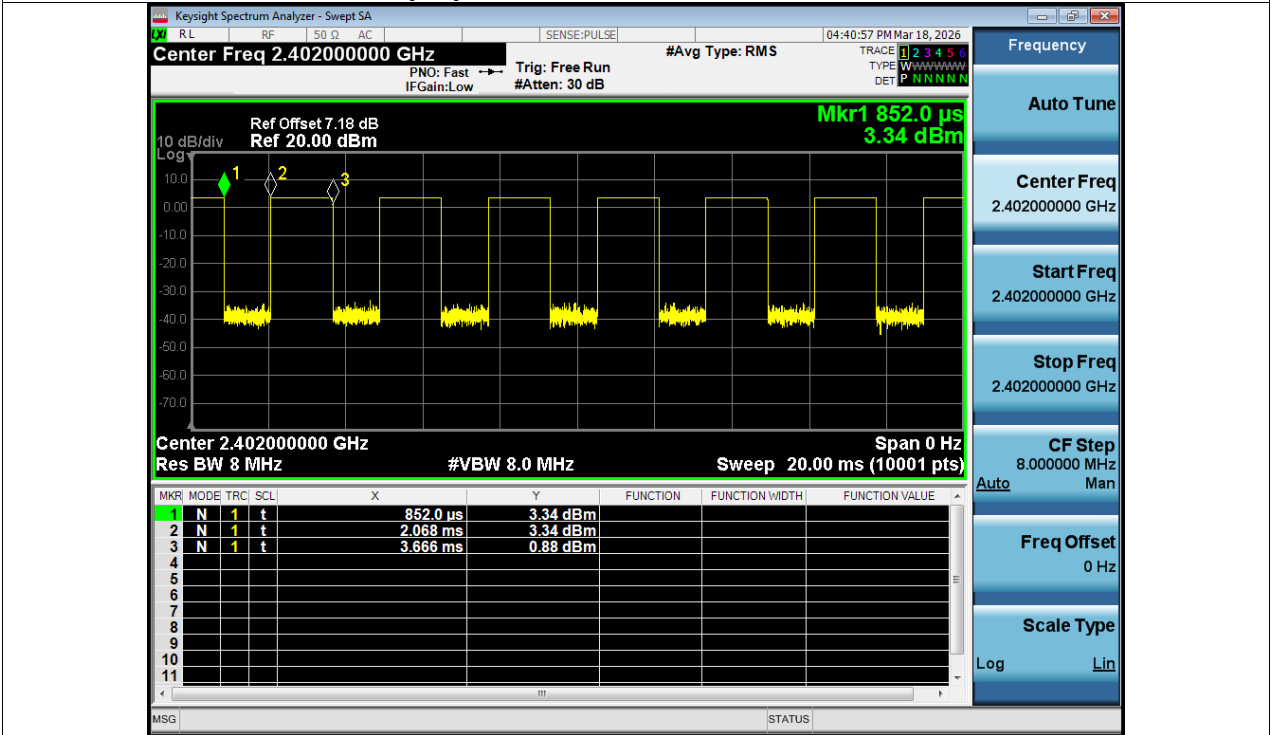
Duty Cycle NVNT BLE 2M 2402MHz Ant1
