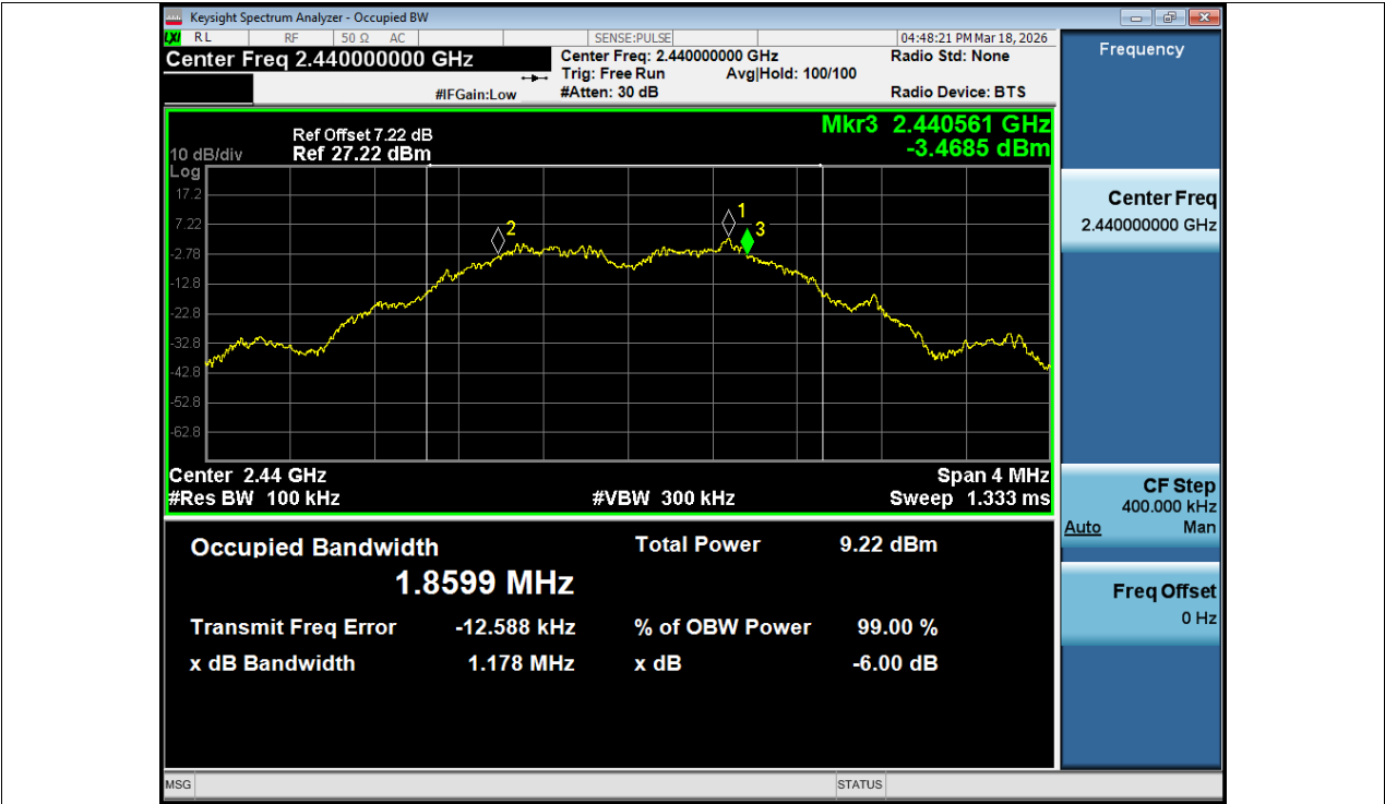
-6dB Bandwidth NVNT BLE 2M 2440MHz Ant1
