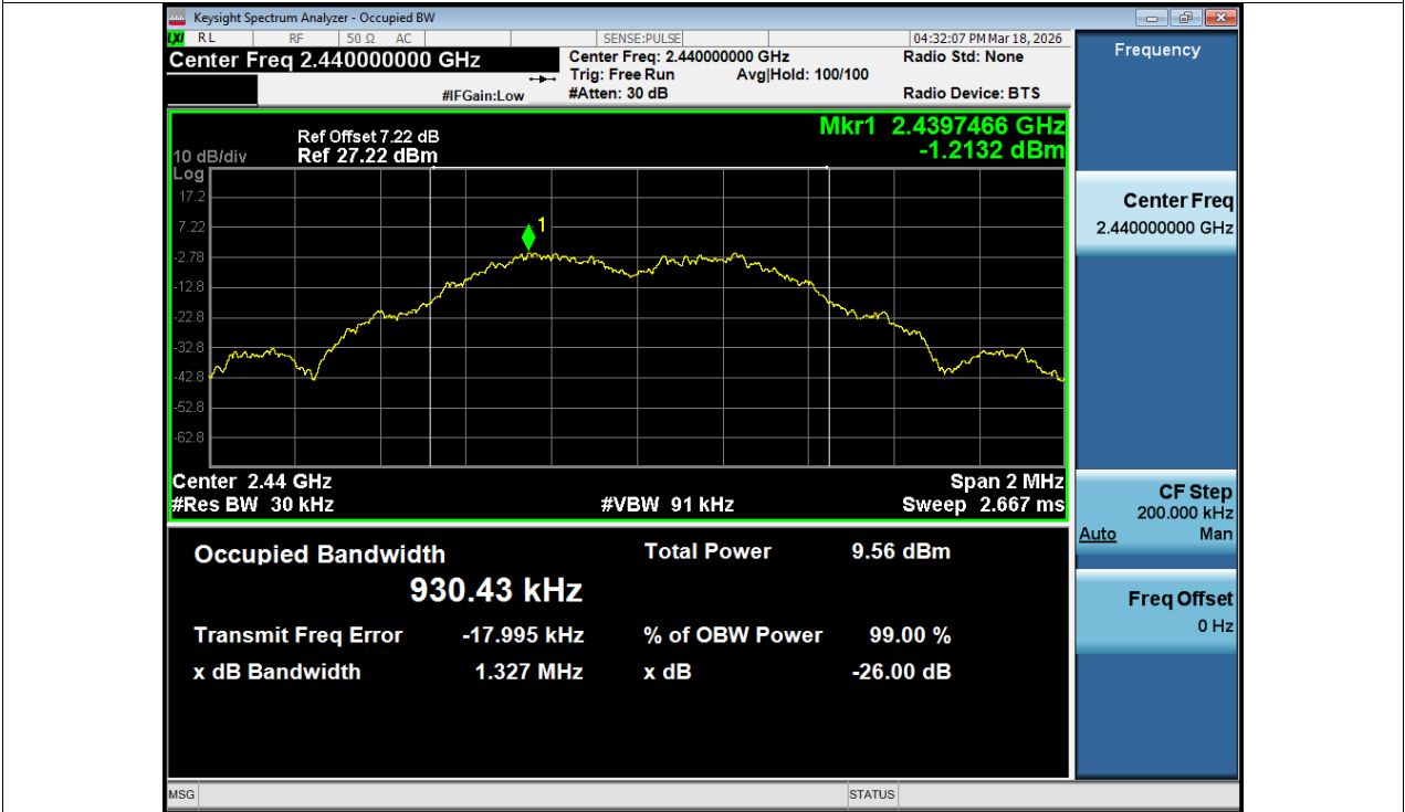
OBW NVNT BLE 1M 2440MHz Ant1
