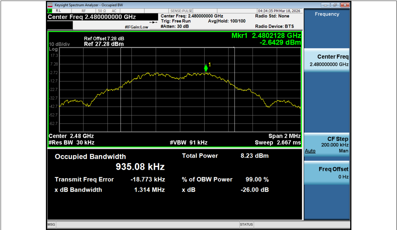
OBW NVNT BLE 1M 2480MHz Ant1
