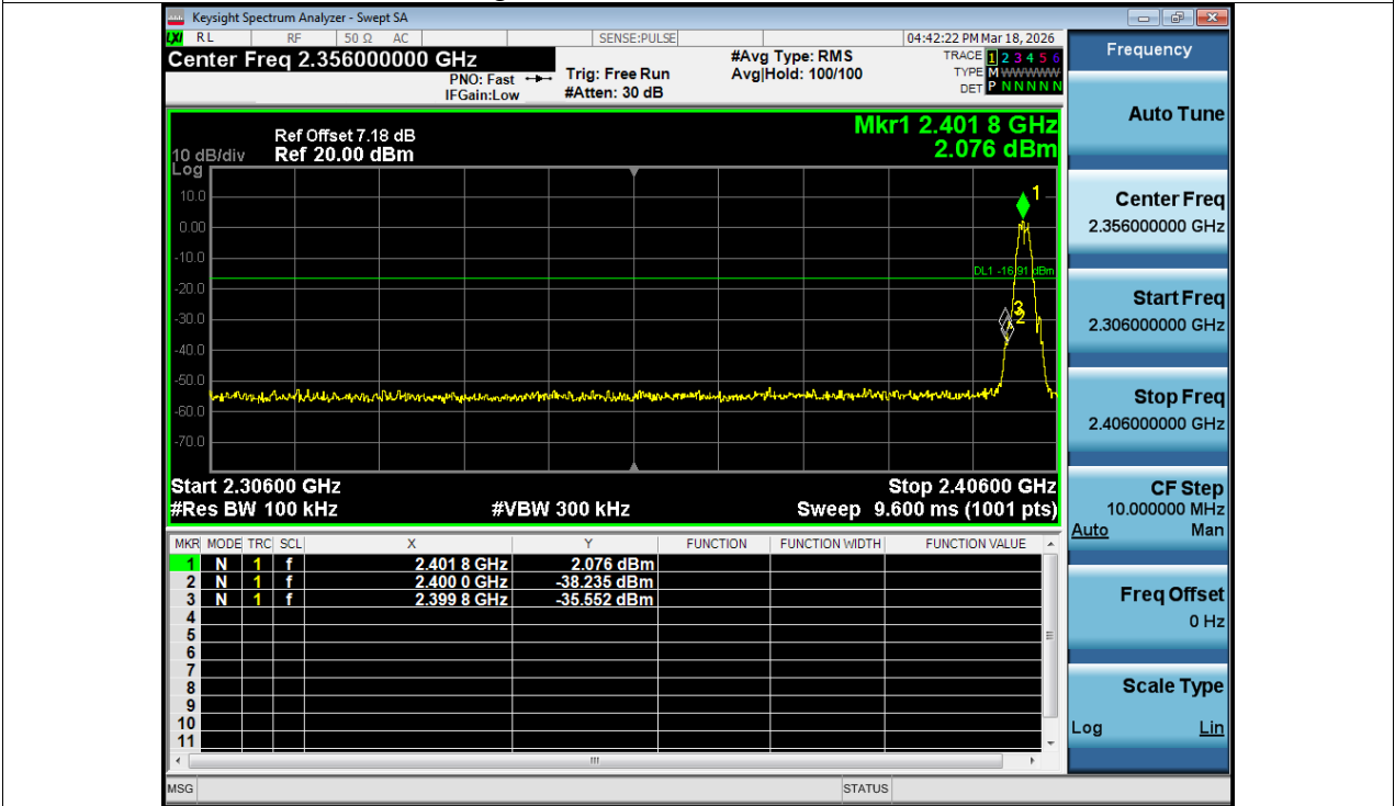
Band Edge NVNT BLE 2M 2402MHz Ant1 Emission
