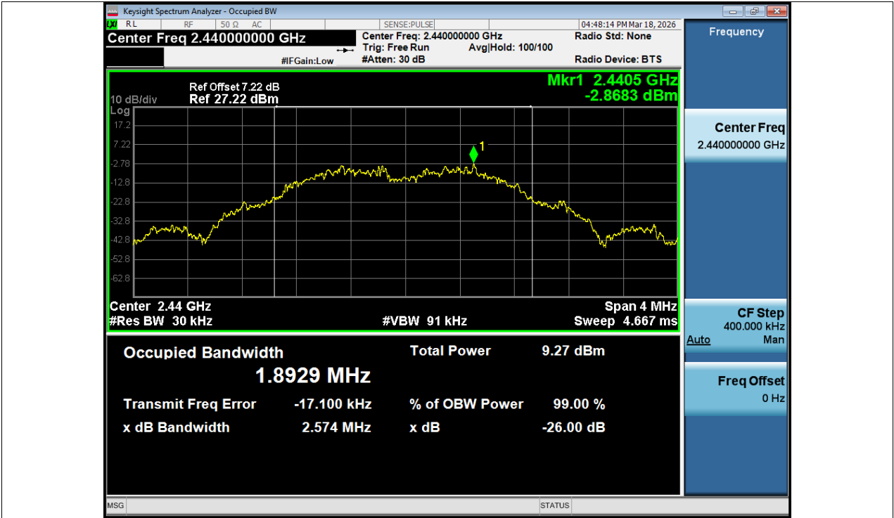
OBW NVNT BLE 2M 2440MHz Ant1
