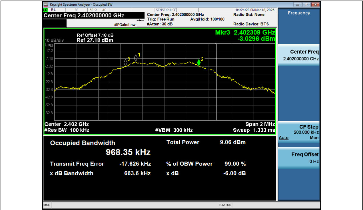
-6dB Bandwidth NVNT BLE 1M 2402MHz Ant1
