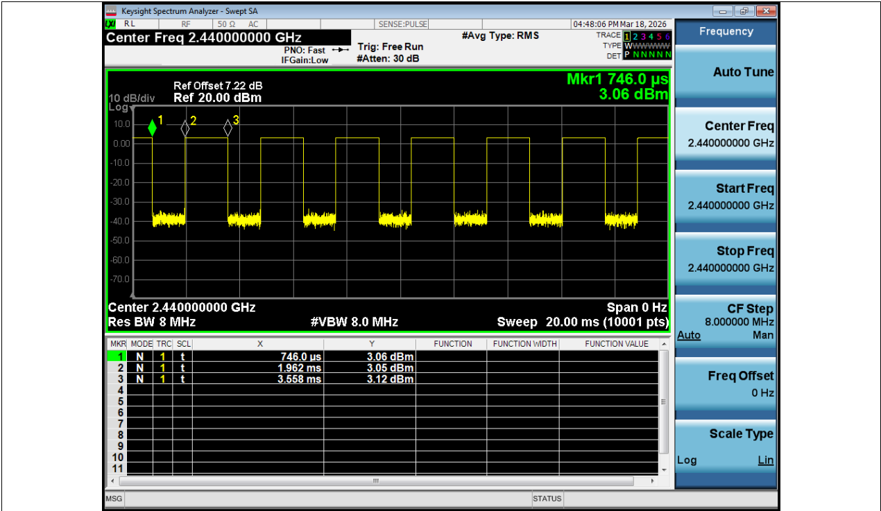
Duty Cycle NVNT BLE 2M 2440MHz Ant1
