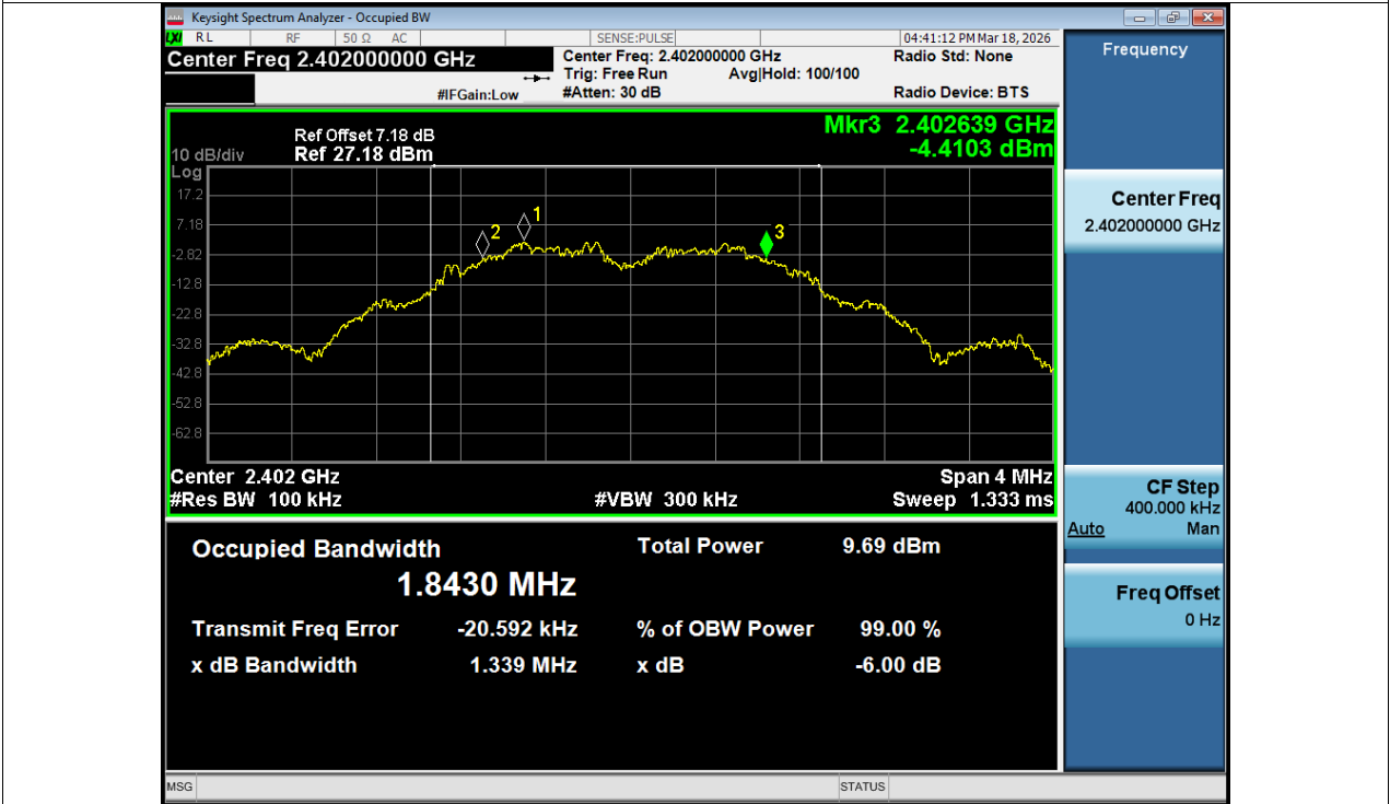
-6dB Bandwidth NVNT BLE 2M 2402MHz Ant1
