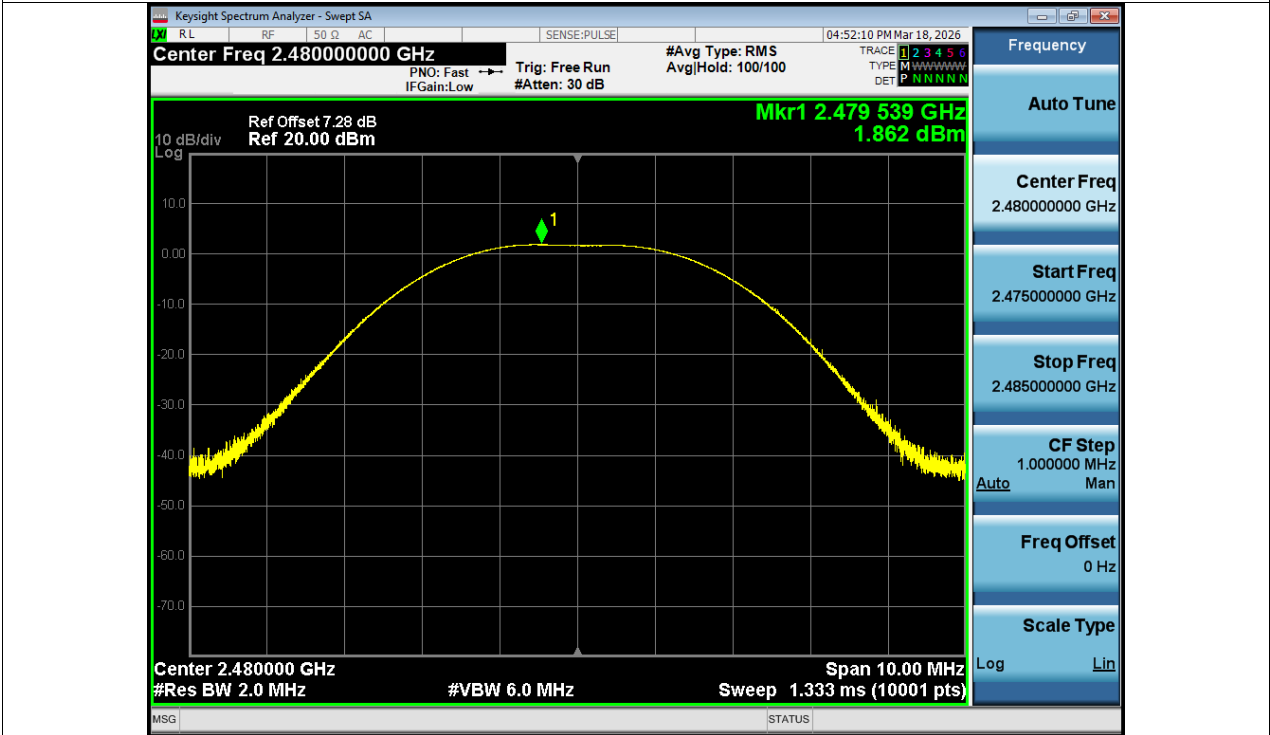
Peak Power NVNT BLE 2M 2480MHz Ant1
