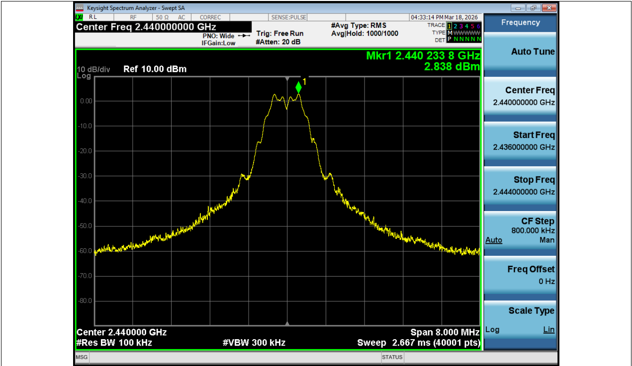
Tx. Spurious NVNT BLE 1M 2440MHz Ant1 Ref
