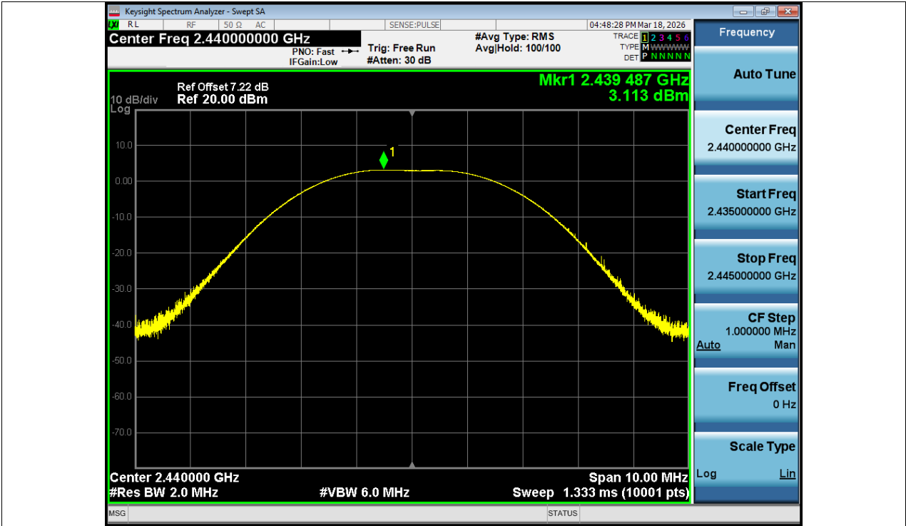
Peak Power NVNT BLE 2M 2440MHz Ant1
