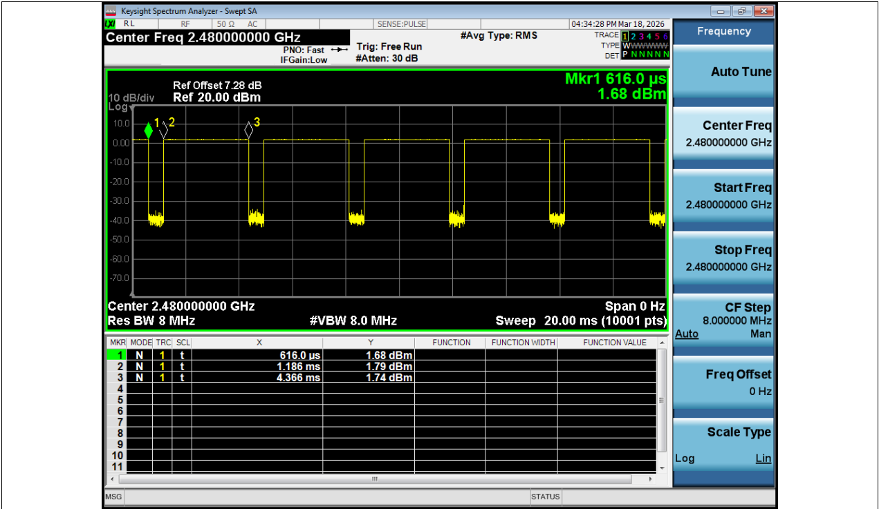
Duty Cycle NVNT BLE 1M 2480MHz Ant1
