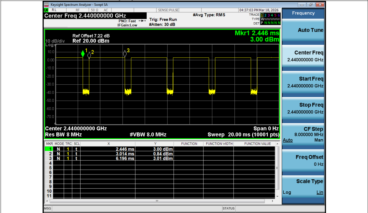
Duty Cycle NVNT BLE 1M 2440MHz Ant1
