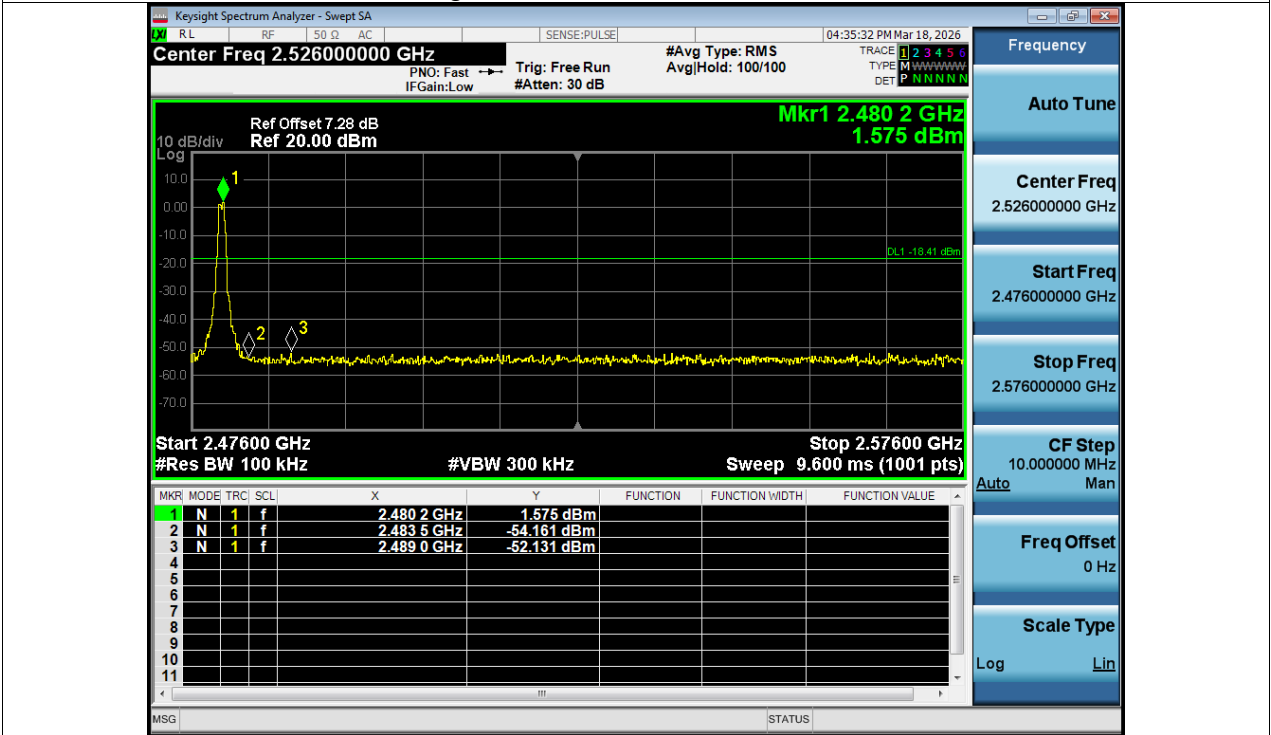
Band Edge NVNT BLE 1M 2480MHz Ant1 Emission
