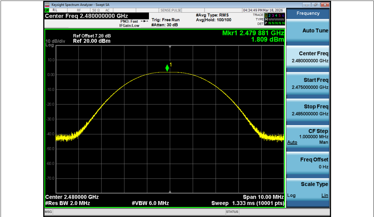
Peak Power NVNT BLE 1M 2480MHz Ant1
