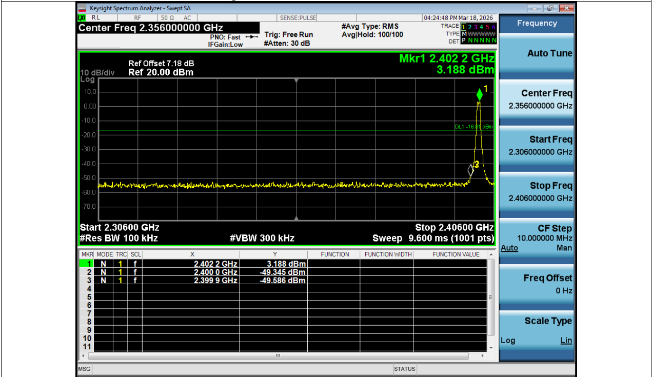
Band Edge NVNT BLE 1M 2402MHz Ant1 Emission
