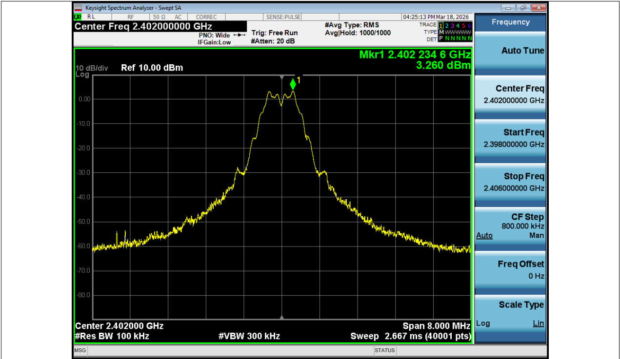
Tx. Spurious NVNT BLE 1M 2402MHz Ant1 Ref
