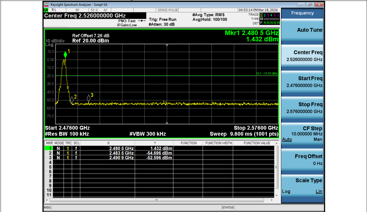
Band Edge NVNT BLE 2M 2480MHz Ant1 Emission
