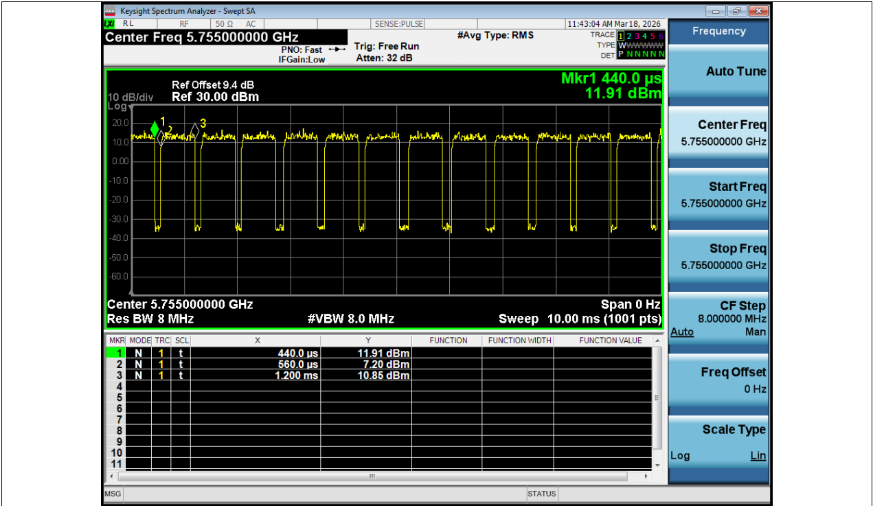
Duty Cycle NVNT n40 5755MHz Ant1
