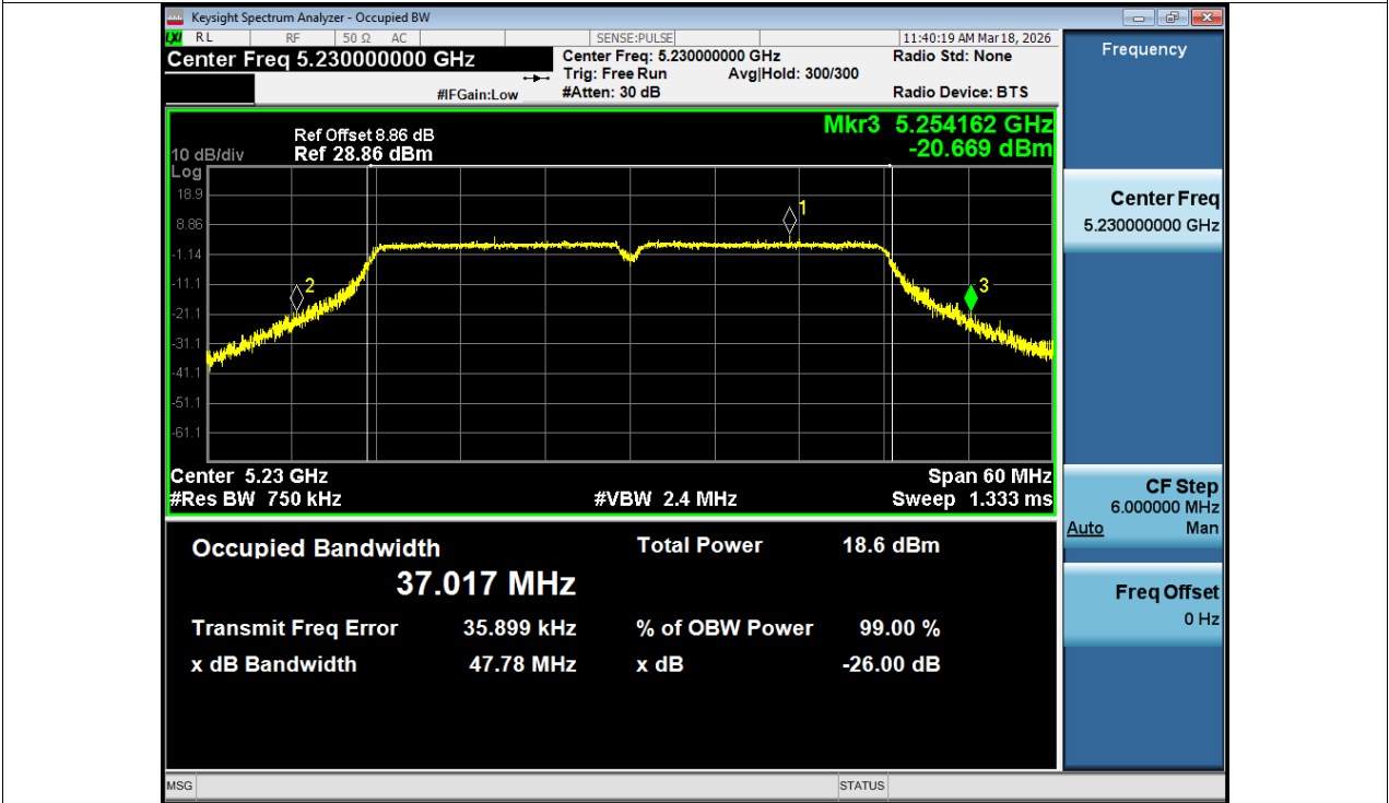
-26dB Bandwidth NVNT n40 5230MHz Ant1
