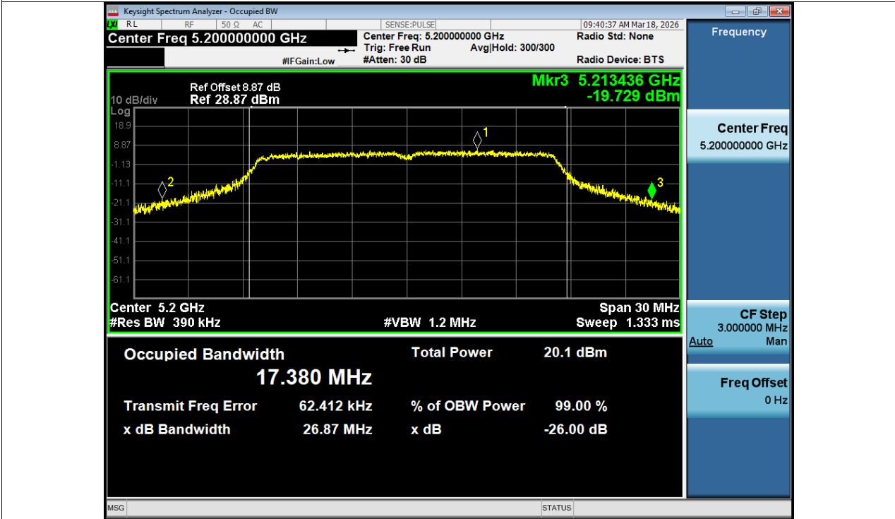
-26dB Bandwidth NVNT a 5200MHz Ant1
