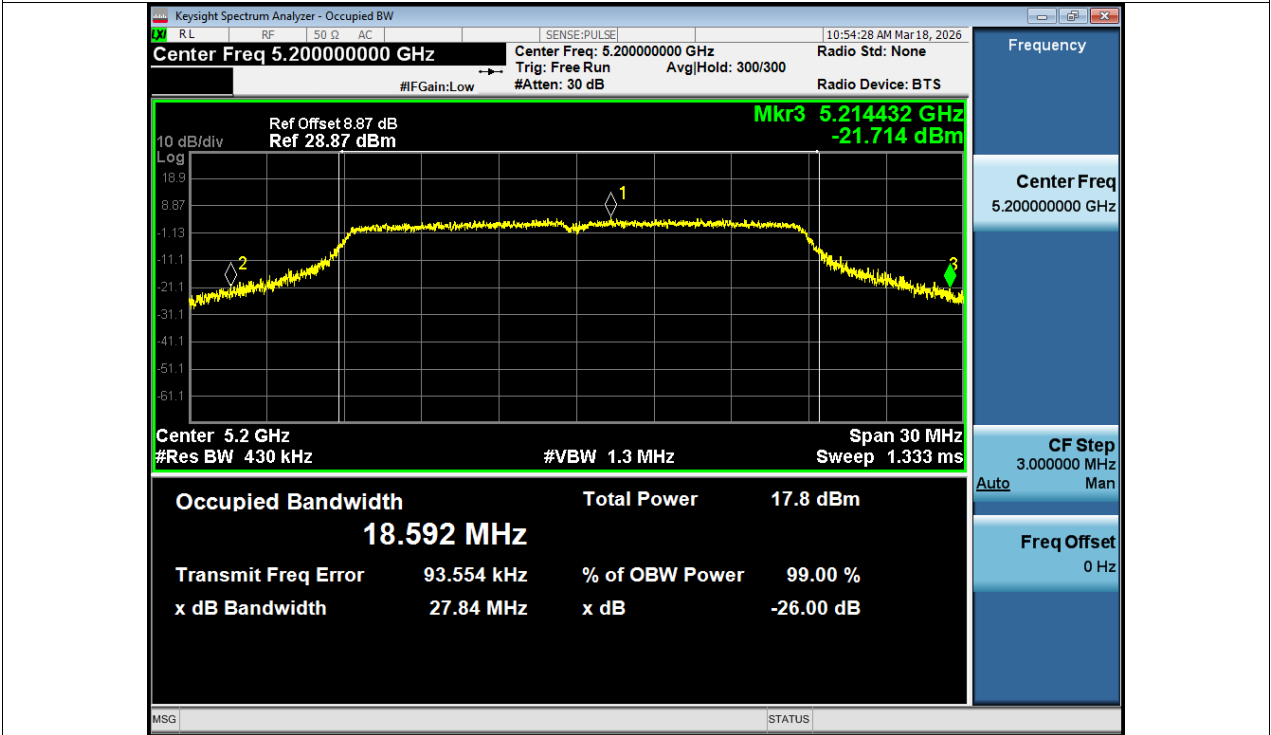
-26dB Bandwidth NVNT ac20 5200MHz Ant1
