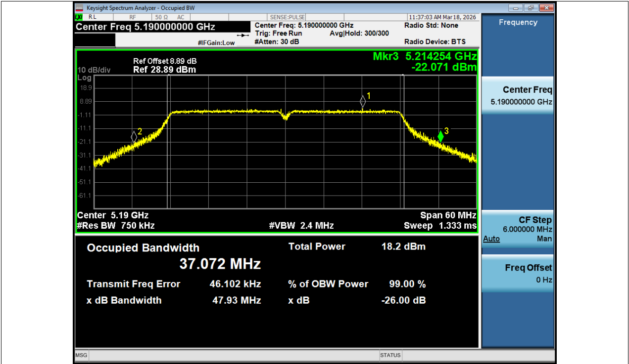
-26dB Bandwidth NVNT n40 5190MHz Ant1
