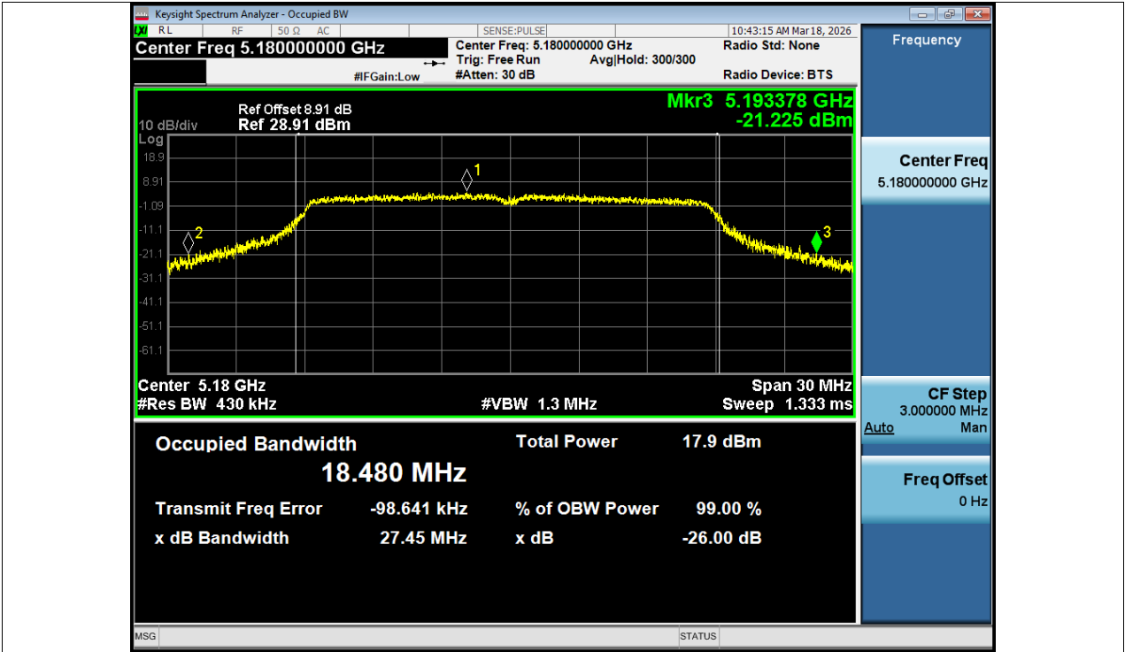
-26dB Bandwidth NVNT ac20 5180MHz Ant1
