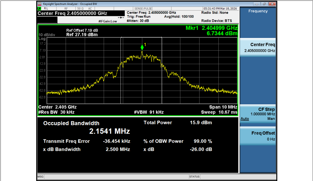
OBW NVNT Zigbee 2405MHz Ant1
